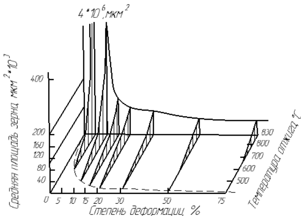
Рис. 2.9. Диаграмма рекристаллизации электролитического железа. Исходная обработка: ковка и отжиг при 930°С; окончательная обработка: холодное осаживание и отжиг 1 ч (Обергоффер, Ортель)
