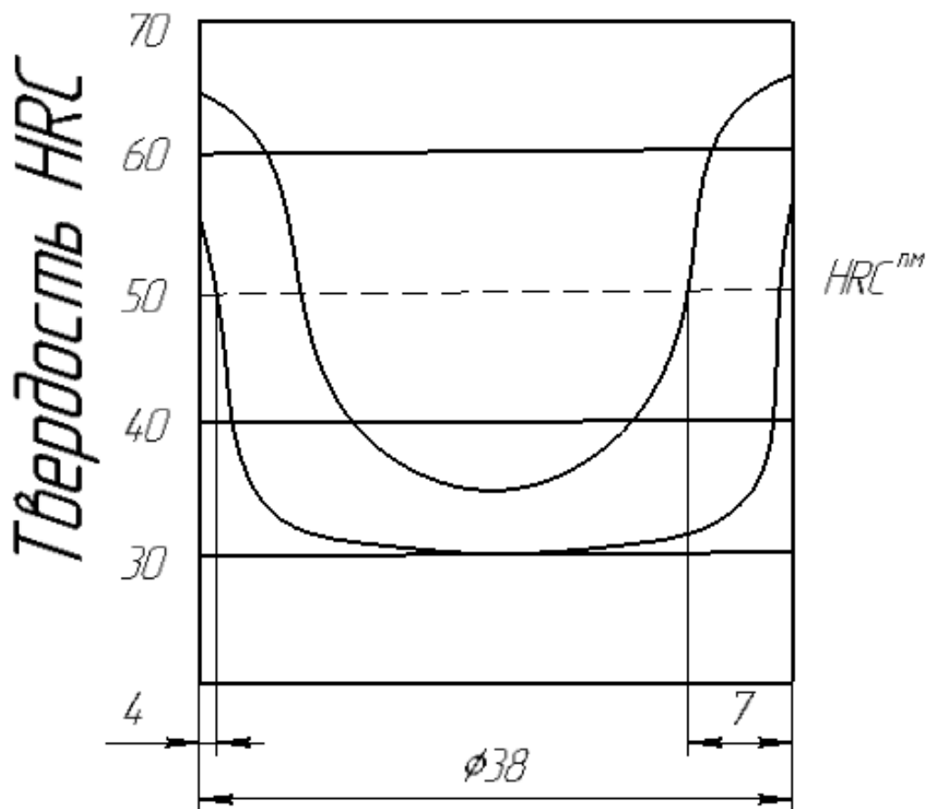
Рис. 4.18. Распределение твердости по диаметру образца из стали 60, закаленного с 815°C: 1 – закалка в воде; 2 – закалка в масле; HRC^{PM} – твердость стали с полумартенситной структурой
