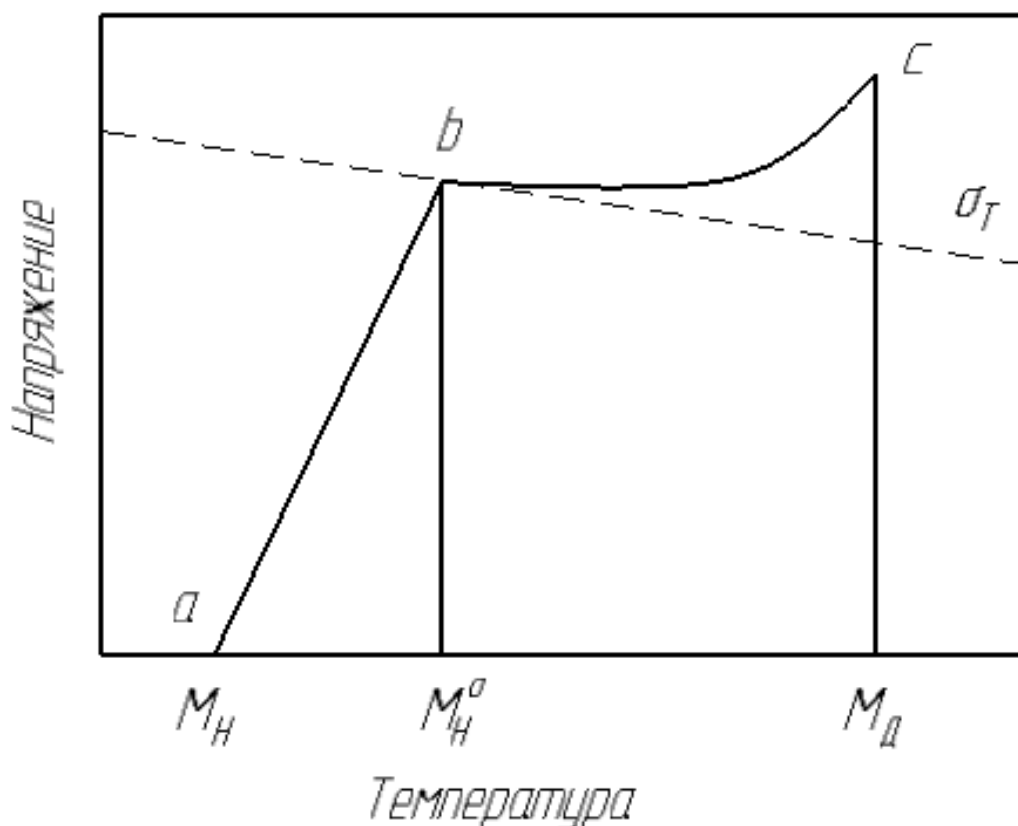
Рис. 4.11. Напряжения, вызывающие мартенситное превращение при упругой деформации (участок ab ) в интервале M_n - M_n^\sigma и при пластической деформации (участок bc ) в интервале M_n^\sigma - M_d (схема по Олсону и Коэну)
