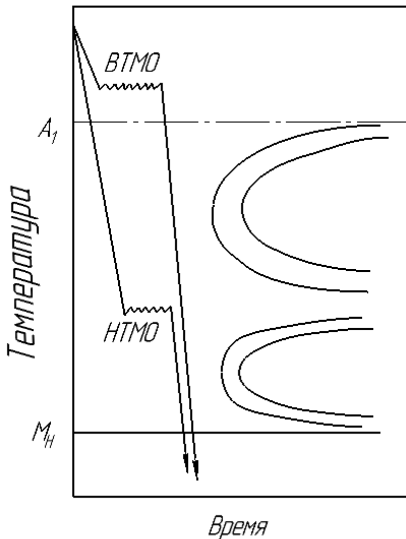
Рис. 6.1. Схема высокотемпературной (ВТМО) и низкотемпературной (НТМО) термохимической обработки легированной стали, закаливаемой на мартенсит
