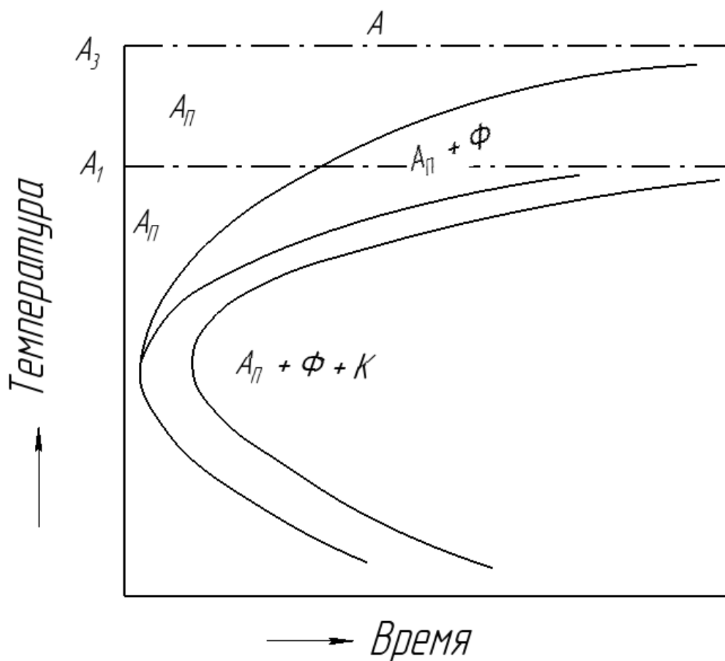
Рис. 3.8. Диаграмма изотермического распада аустенита в доэвтектоидной стали (схема): А – устойчивый аустенит; A_{п} – переохлажденный аустенит; Ф – феррит; К – карбид
