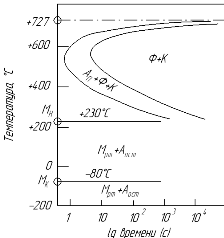
Рис. 4.2. C-диаграмма с мартенситными точками для стали с 0,8% C:
