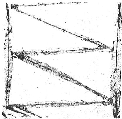
Рис. 4.8. Фермообразное расположение пластин мартенсита и остаточный аустенит (светлый фон) в закаленной стали с 1,66% С. х550 (Краус и Мадер)
