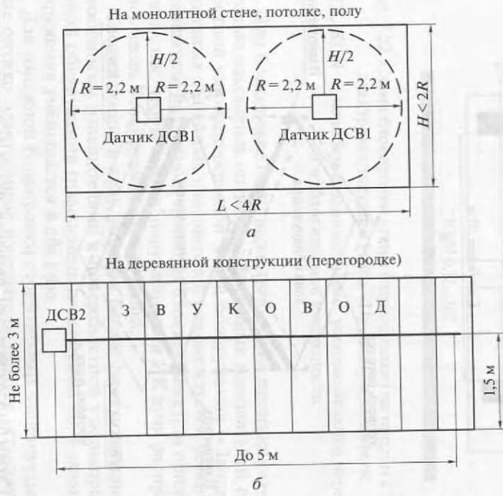
Рис. 7.24. Схемы блокировки стен, потолков, полов (а), деревянных конструкций (б) на разрушение с помощью пьезоэлектрических извещателей
