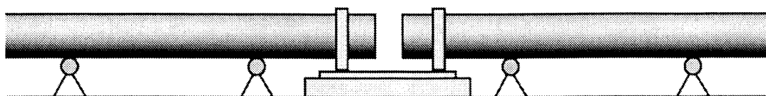
Рис 4.2.10 Правильное положение труб при сварке достигается с помощью специальных опор
