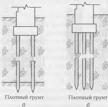
Рис. 8.5. Свайные фундаменты: а — сваи-стойки; б — висячие сваи
