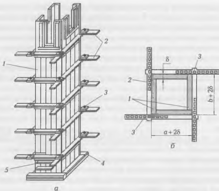
Рис. 11.2. Опалубка колонны:
