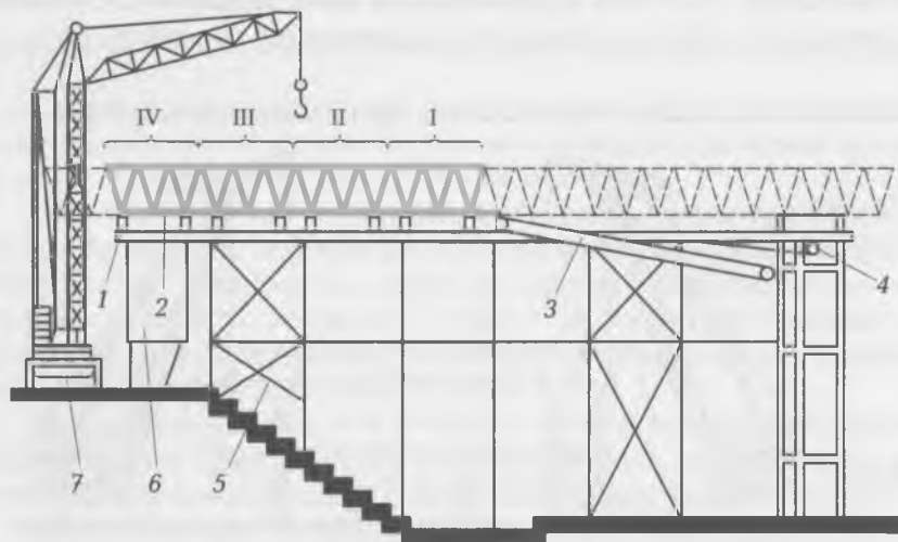
Рис. 10.5. Монтаж структурного покрытия движкой с наращиванием:
