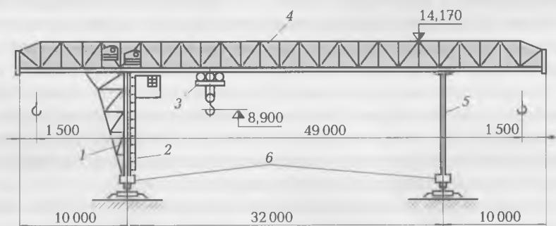
Рис. 6.2. Козловой кран:
