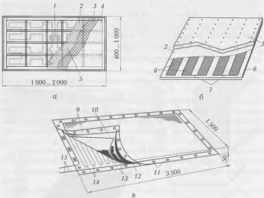
Рис. 11.10.Греющая (термоактивная) опалубка:
