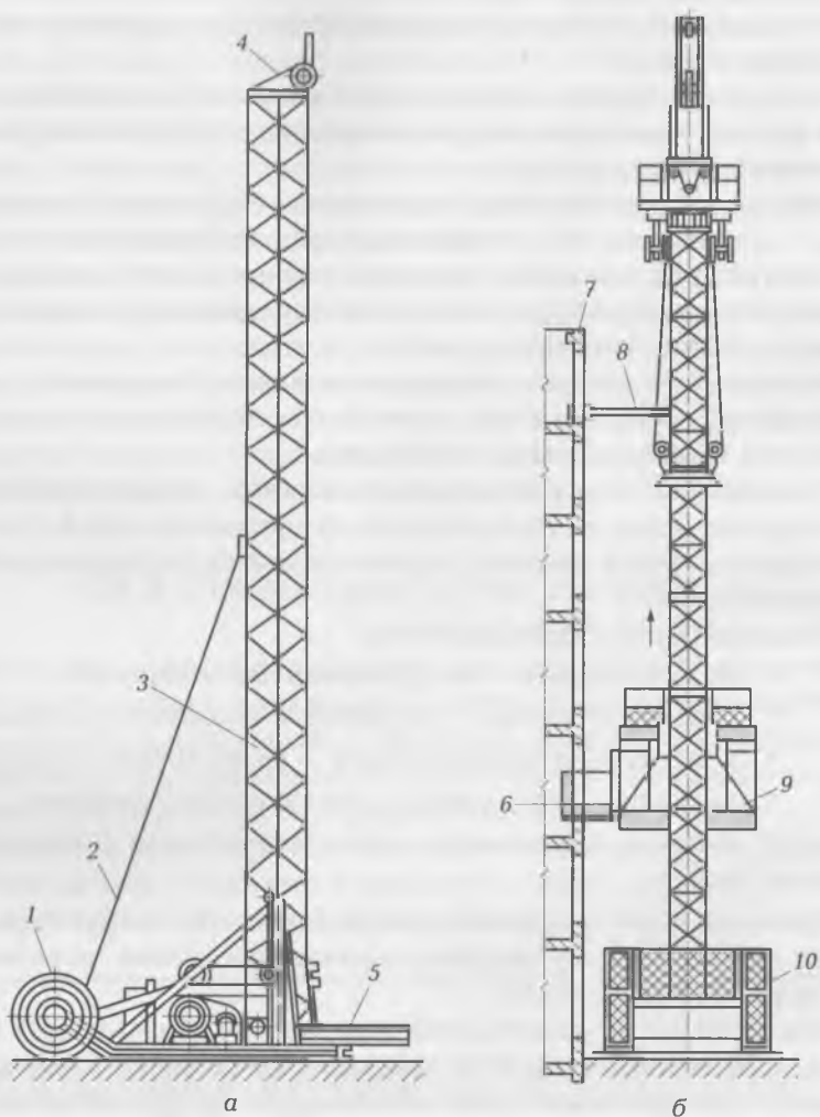
Рис. 6.3. Мачтовые подъемники:
