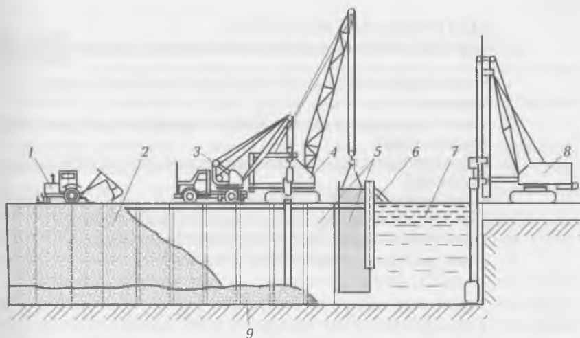
Рис. 8.16. Возведение «стены в грунте» из сборных железобетонных плит:
