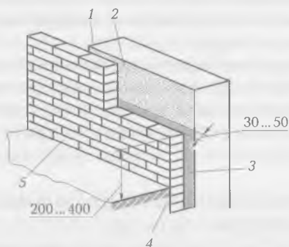
Рис. 15.1. Устройство вертикальной литой асфальтовой гидроизоляции:
