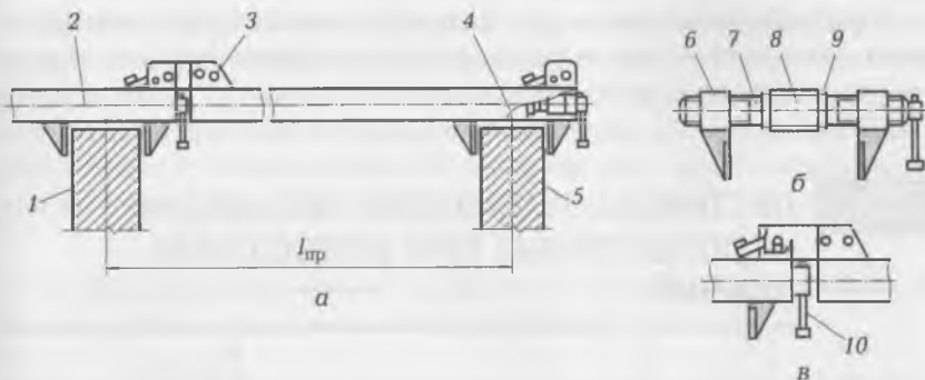
Рис. 6.24. Горизонтальная связь для фиксации панелей по геометрическим осям: a — общий вид; б — трубка; в — узел соединения связей; 1, 5 — панели; 2 — корпус; 3 — замок; 4 — осевой фиксатор; 6 — наружная втулка с прижимом; 7 — шпилька с левой и правой резьбой; 8 — втулка; 9 — упорное кольцо; 10 — вороток; l_{пр} — длина пролета
