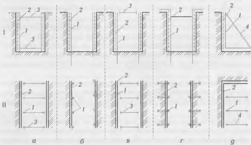
Рис. 4.5. Схемы крепления вертикальных стенок выемок:
