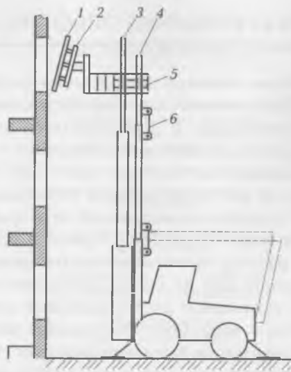
Рис. 16.2. Установка витринного стекла:
