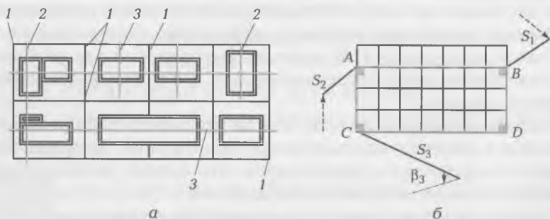
Рис. 3.1. Строительная сетка:
