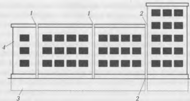
Рис. 1.4. Схемы размещения и конструкция деформационных швов: 1 — температурный шов; 2 — осадочный шов; 3 — фундамент; 4 — стена
