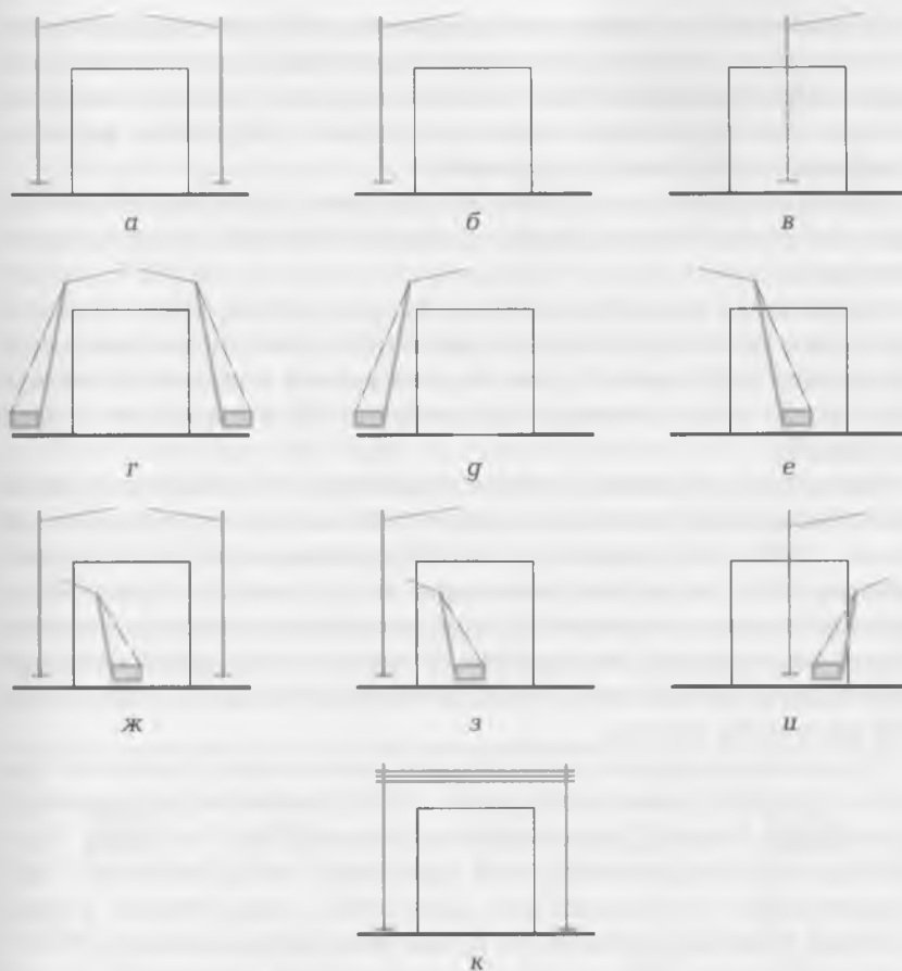
Рис. 9.1. Варианты расстановки кранов:
