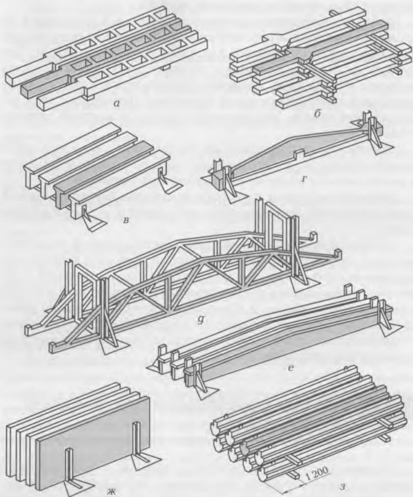
Рис. 5.4. Складирование железобетонных конструкций промышленных зданий: а — колонн одноэтажных зданий; б — колонн многоэтажных зданий; в — подкрановых балок; г — подстропильных балок; д — стропильных ферм; е — стропильных балок; ж — стеновых панелей; з — ригелей
