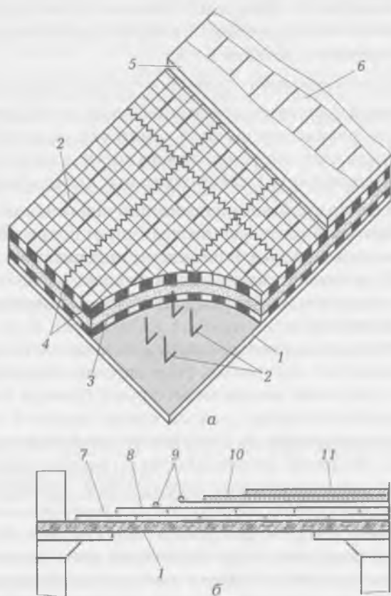
Рис. 15.2. Теплоизоляция из рулонных материалов и сборных плит: а — обволакивающая теплоизоляция; б — сборно-блочная теплоизоляция; 1 — изолируемая поверхность; 2 — шпильки; 3 — минераловатные маты; 4 — сетки; 5 — штукатурка; 6 — оклейка; 7 — плиты первого слоя; 8 — плиты второго слоя; 9 — слой пергамина; 10 — железобетонная плита; 11 — чистый пол
