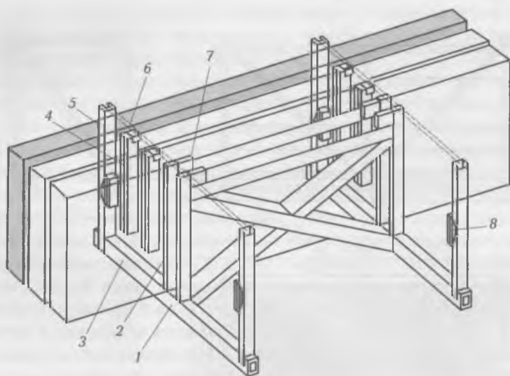
Рис. 5.3. Контейнер для стеновых панелей:
