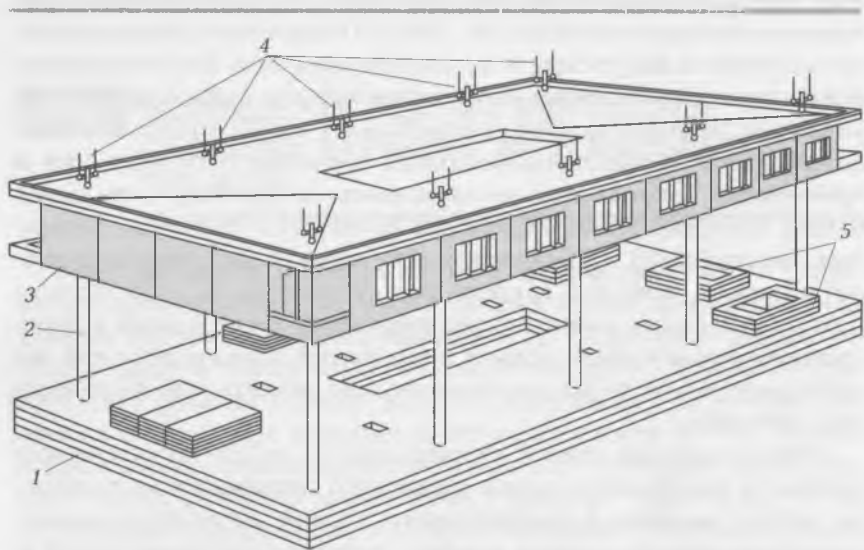
Рис. 9.5. Схема возведения зданий методом подъема этажей: 1 — пакет плит перекрытий; 2 — колонны; 3 — стеновые панели; 4 — домкраты; 5 — сборные элементы
