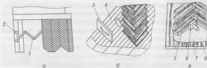
Рис. 16.9. Настилка полов из штучного паркета:
