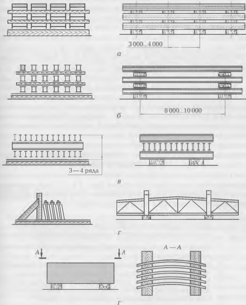
Рис. 5.5. Складирование стальных конструкций:
