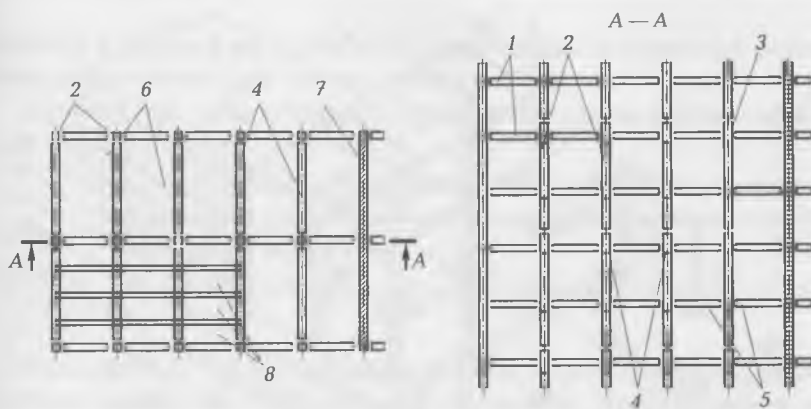
Рис. 1.11. Каркас здания с полной каркасной системой:
