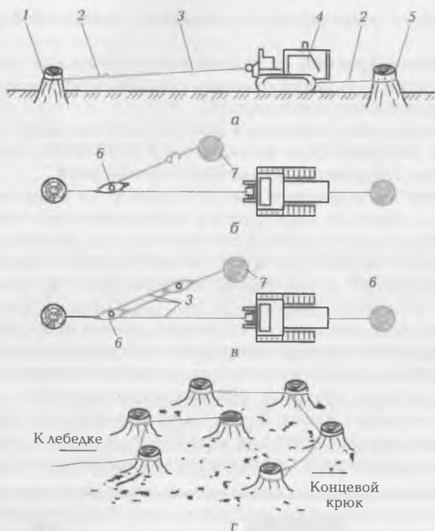
Рис. 3.5. Корчевка пней тракторной трелевочно-корчевальной лебедкой:
