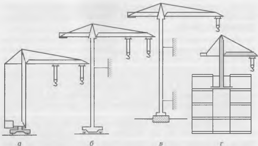
Рис. 6.1. Виды башенных кранов:
