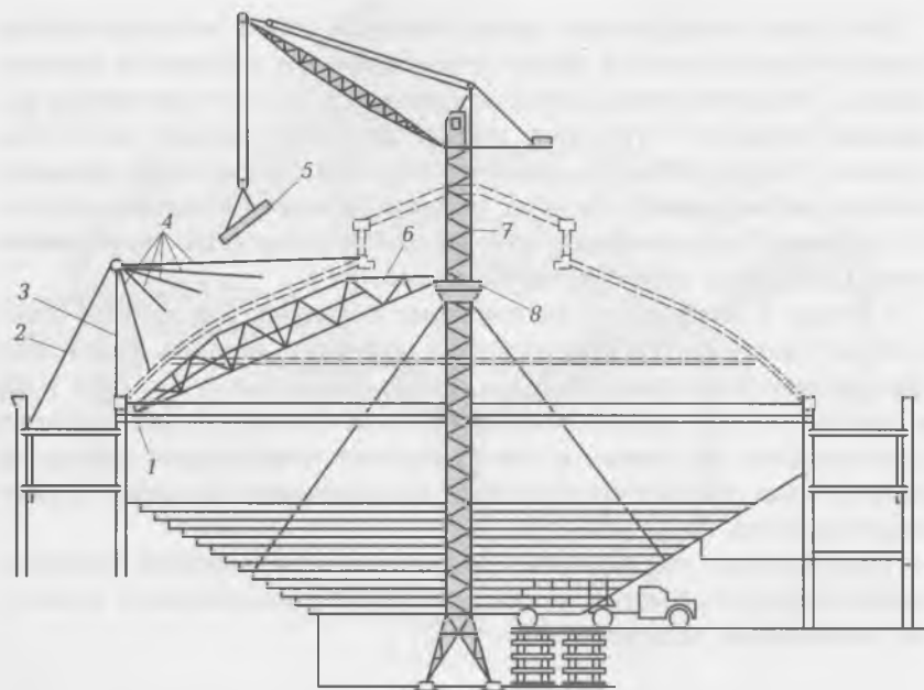
Рис. 9.15. Схема монтажа купольного покрытия:
