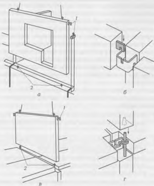
Рис. 9.10. Установка внутренних и наружных стеновых панелей методом самофиксации: а — установка наружной стеновой панели; б — фиксатор боковой; в — установка внутренней стеновой панели; г — схема нижней торцевой фиксации; 1 — фиксаторы боковые; 2 — фиксаторы нижние торцевые
