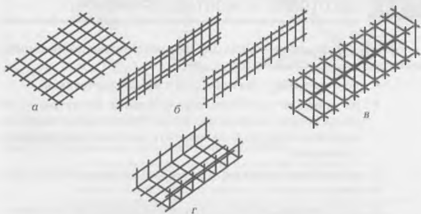
Рис. 11.11. Арматурные элементы:
