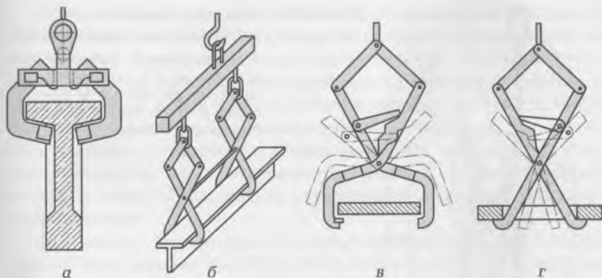
Рис. 6.13. Клещевые захваты для подъема:
