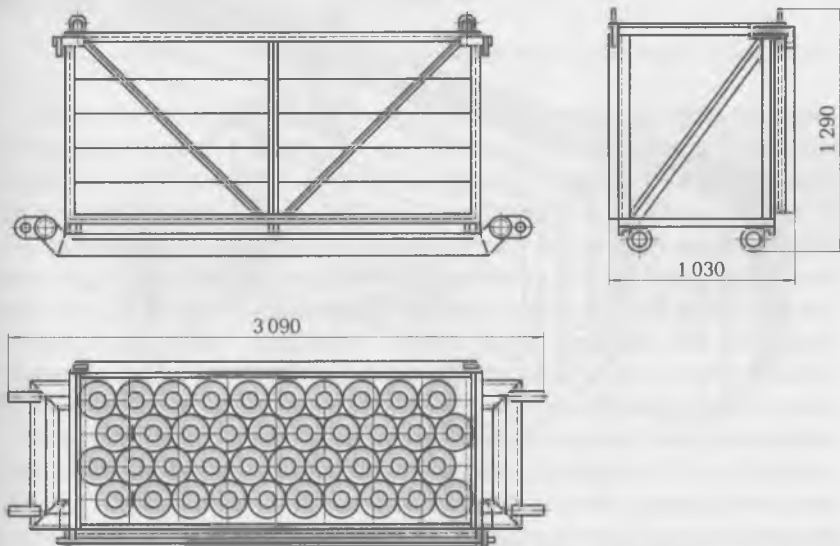
Рис. 5.1. Контейнер грузоподъемностью 1 100 кг для подъема 40 рулонов кровельных материалов
