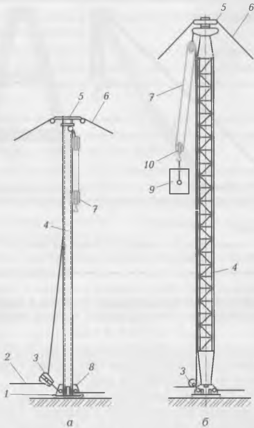
Рис. 6.4. Монтажные мачты:
