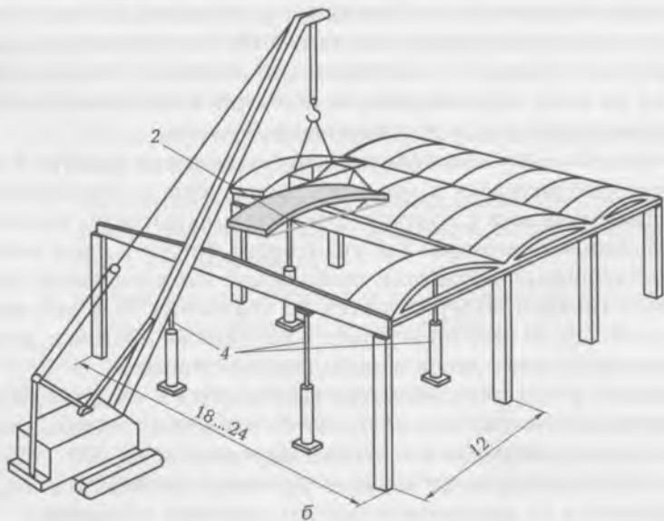
Рис. 9.14. Схемы установки оболочек с опиранием на несущие конструкции: а — двоякой кривизны; б — цилиндрические; 1 — контурные элементы; 2 — временные монтажные затяжки; 3 — готовые секции оболочек; 4 — монтажные временные опоры [размеры указаны в м]
