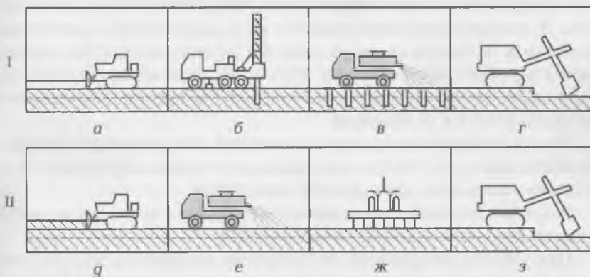
Рис. 4.22. Схемы разработки с химическим оттаиванием грунта: I — с использованием жидкого химического реагента; II — с предварительным «засолением» грунта; а — удаление снежного покрова; б — бурение шпуров; в — разлив раствора химического реагента; г — разработка грунта; д — снятие растительного слоя; е — рассыпание соли; ж — боронование грунта; з — разработка грунта
