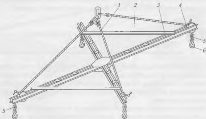
Рис. 9.6. Балансирная траверса для монтажа объемных элементов (блоков-комнат):
