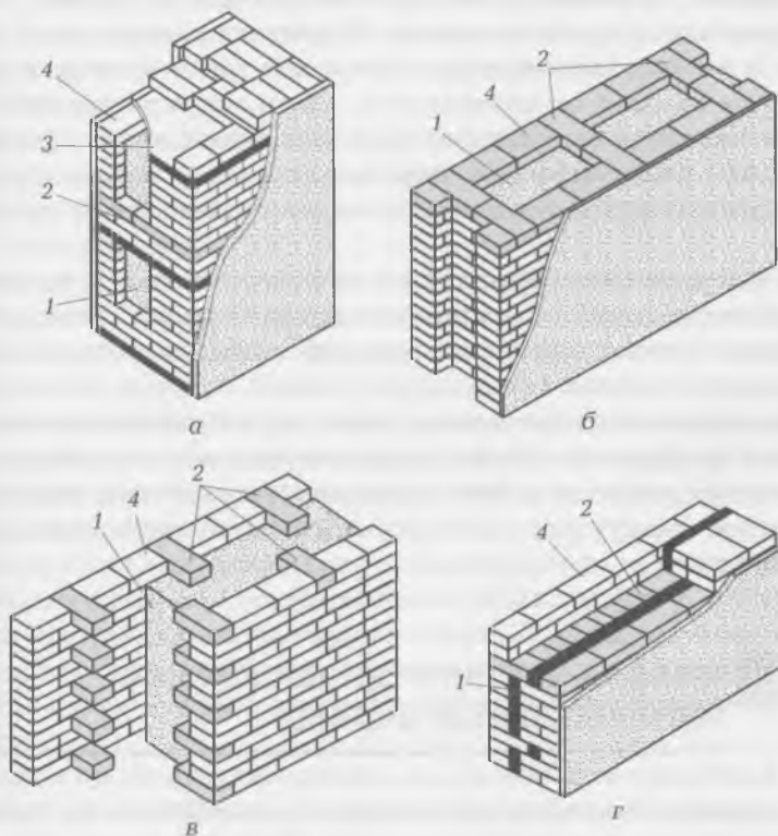
Рис. 12.11. Виды облегченных кирпичных кладок:
