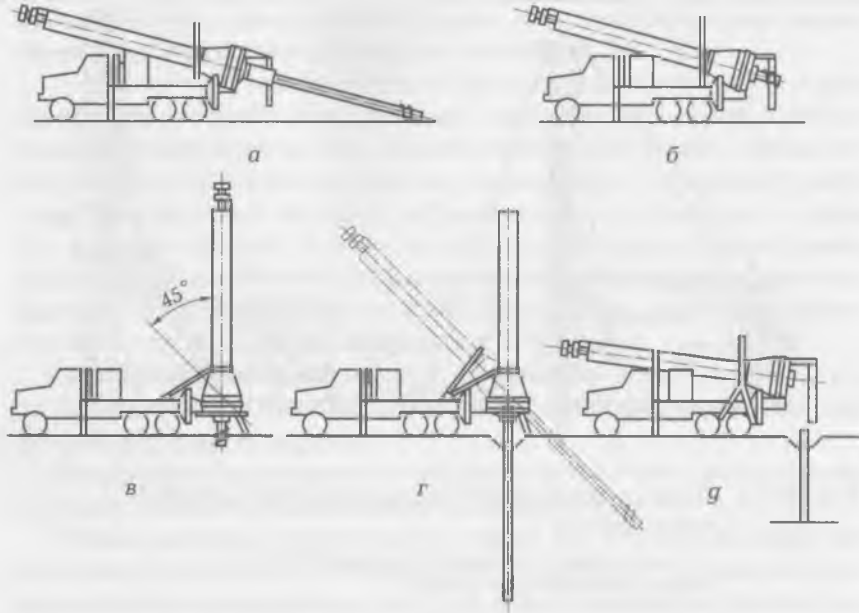
Рис. 8.13. Погружение свай методом завинчивания:
