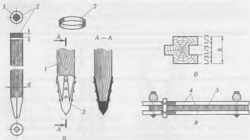
Рис. 8.6. Деревянные шпунт и сваи:
