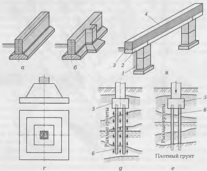
Рис. 1.3. Фундаменты:
