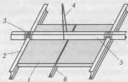
Рис. 1.8. Подвесной потолок: 1 — плита; 2 — алюминиевый профиль; 3 — хомут; 4 — подвеска; 5 — несущий стальной профиль; 6 — стальная шпонка
