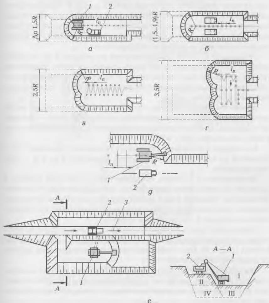
Рис. 4.8. Схемы экскаваторных проходок с рабочим оборудованием «прямая лопата»: а — лобовая (торцовая) проходка; б — лобовая (торцовая) проходка с двухсторонним расположением транспорта; в — уширенная лобовая проходка с движением экскаватора «зигзаг»; г — поперечно-торцовая проходка; д — боковая проходка; е — разработка котлована по ярусам: I...IV — ярусы разработки; 1 — экскаватор; 2 — автосамосвал; 3 — направление движения транспорта; R — радиус действия; l_n — шаг перестановки (стоянки)
