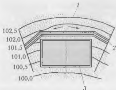
Рис. 3.6. Защита площадки от поступления поверхностных вод: 1 — бассейн стока воды; 2 — нагорная канава; 3 — строительная площадка
