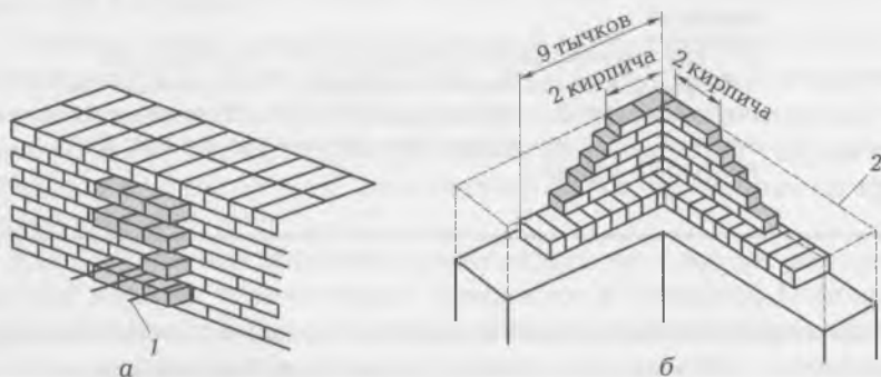
Рис. 12.4. Сопряжение стен с устройством штраб:
