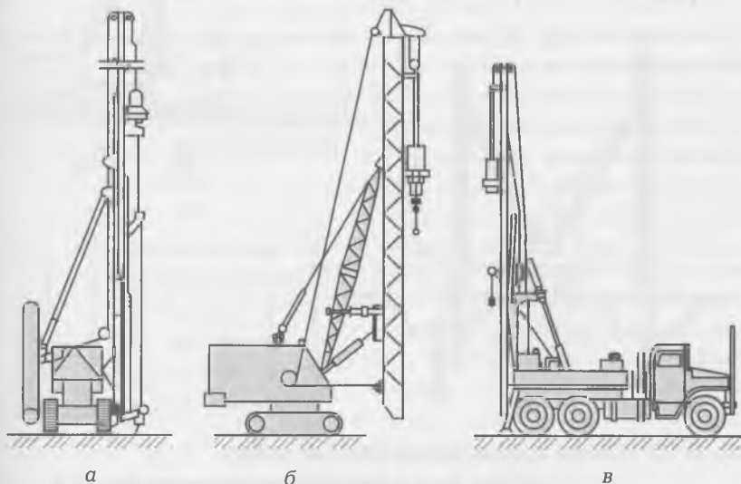
Рис. 8.9. Схемы самоходных сваебойных агрегатов: а — на тракторе; б — на экскаваторе; в — на автомобиле
