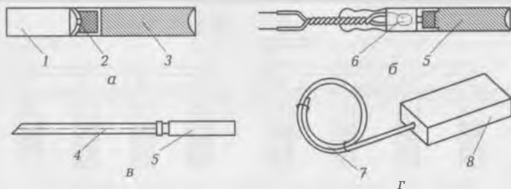
Рис. 4.17. Средства взрывания:
