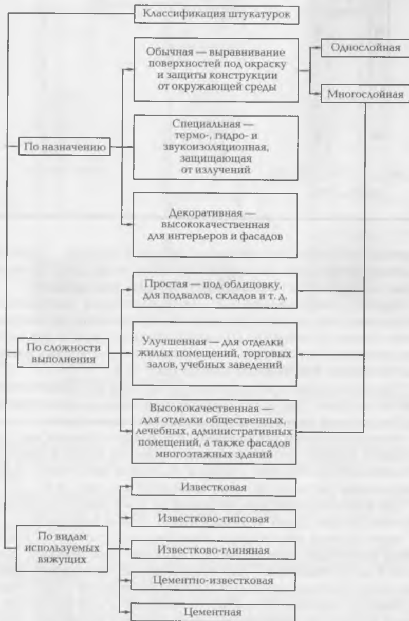
Рис. 16.3. Классификация штукатурок
