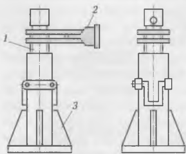
Рис. 6.16. Винтовой домкрат:
