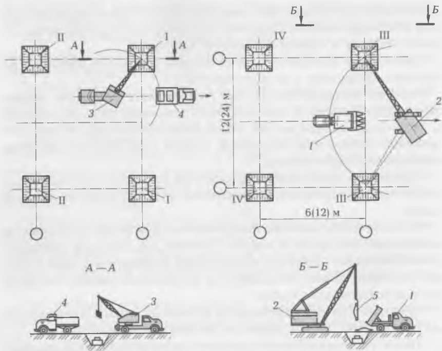
Рис. 8.4. Схема технологического процесса устройства монолитных железобетонных фундаментов с укладкой бетонной смеси с помощью кранов:
