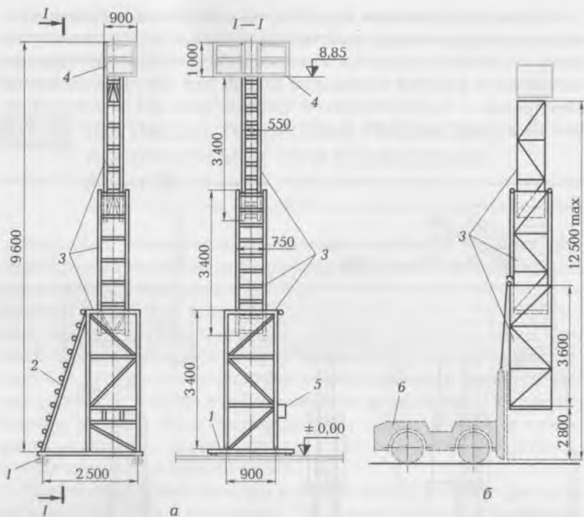
Рис. 6.26. Передвижные телескопические подмости:
