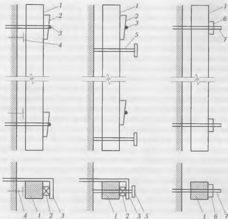
Рис. 16.5. Варианты установки инвентарных маяков (устройство растворных маяков): 1 — правило; 2 — клин; 3 — костыль; 4 — инвентарная марка; 5 — болт; 6 — гайка; 7 — штырь с резьбой
