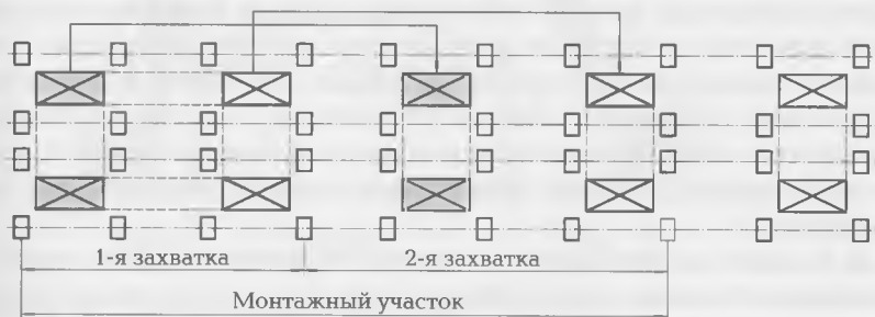
Рис. 9.11. Схема расположения и перестановки кондукторов
