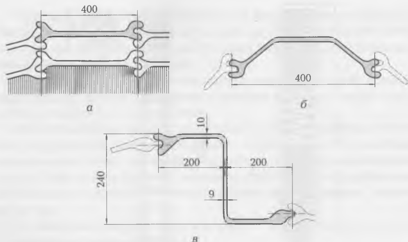
Рис. 8.8. Металлический шпунт: а — плоский; б — корытообразный; в — Z-образный
