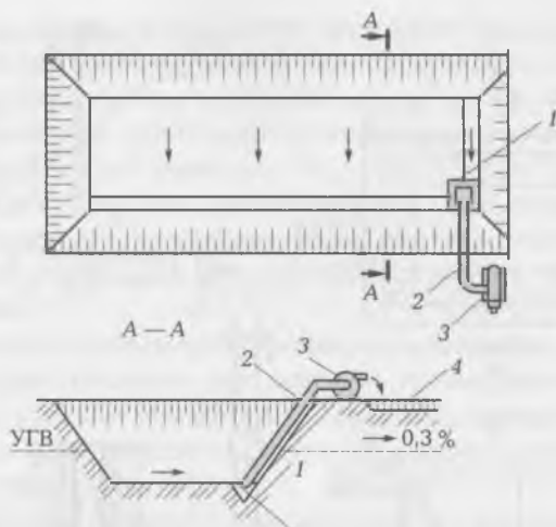
Рис. 4.3. Открытый водоотлив:
