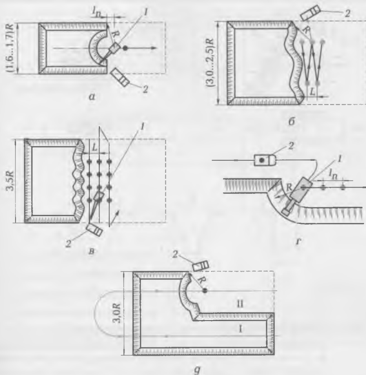
Рис. 4.9. Схемы проходок экскаватора с рабочим оборудованием драглайн и «обратная лопата»: а — лобовая проходка; б — уширенная лобовая проходка; в — поперечно-торцовая проходка; г — боковая проходка; д — разработка котлована двумя лобовыми проходками; 1, II — последовательность проходок; 1 — экскаватор; 2 — автосамосвал; L — расстояние между проходками
