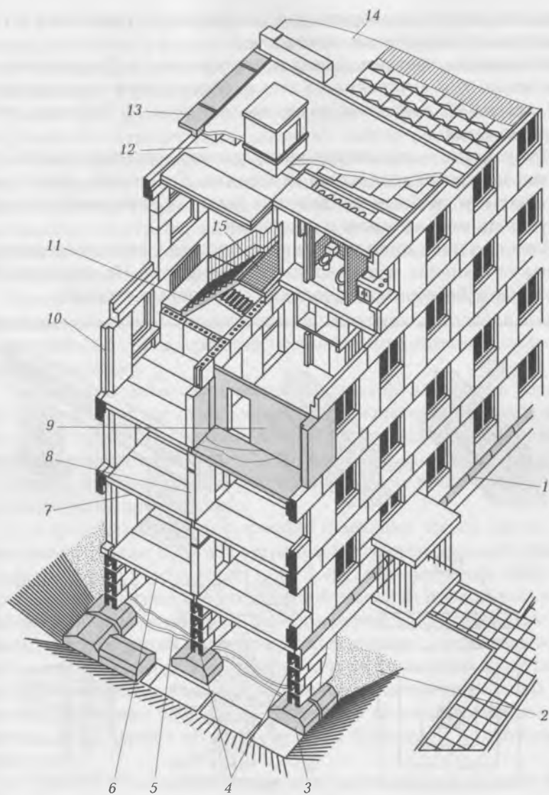
Рис. 1.2. Гражданское здание:
