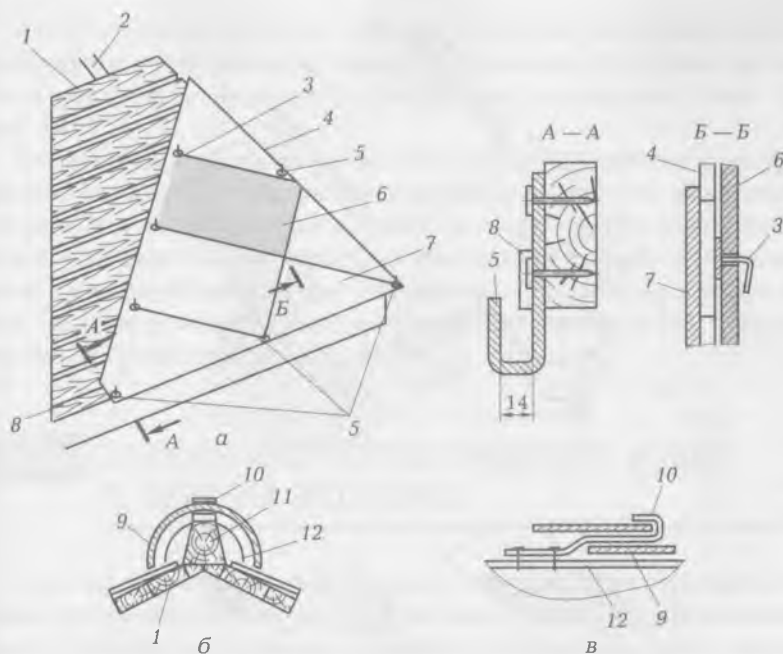
Рис. 14.6. Кровля из асбоцементных плоских плиток:
