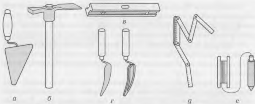
Рис. 12.8. Инструмент для каменных работ:
