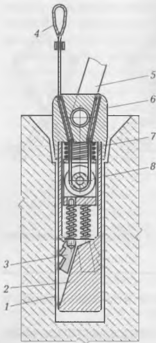
Рис. 6.14. Клиновой захват с дистанционным управлением: 1 — отверстие; 2 — клиновидный наконечник; 3 — кулачки; 4 — канат для расстроповки; 5 — скоба; 6 — оголовок; 7 — пружина; 8 — блок
