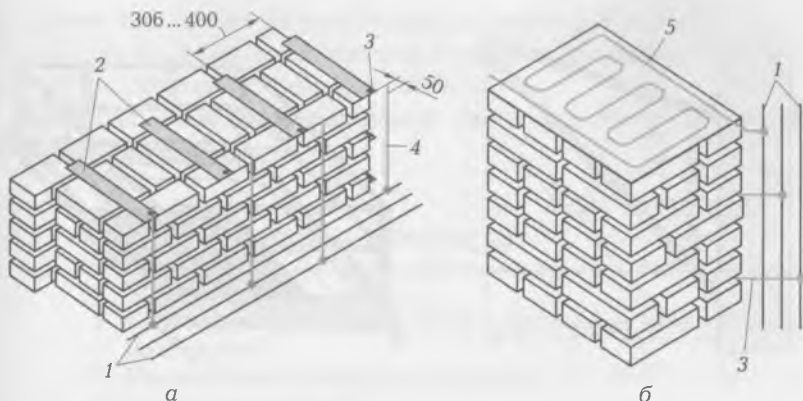
Рис. 12.13. Схемы электропрогрева:
