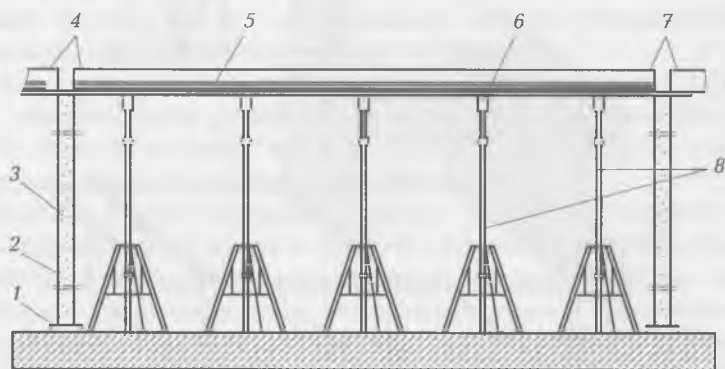
Рис. 11.6. Опалубка балочного перекрытия (разборно-переставная):
