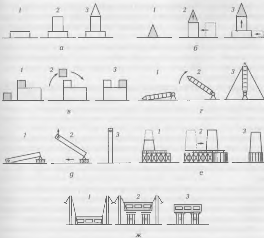
Рис. 7.3. Способы монтажа:
