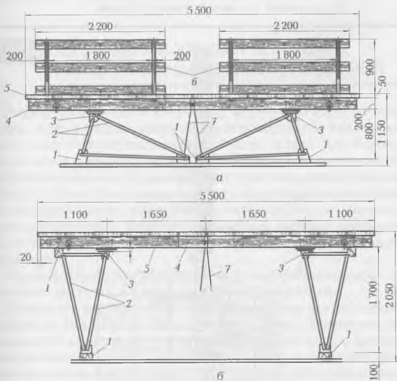
Рис. 12.7. Шарнирно-панельные подмости для каменной кладки: а — при кладке второго яруса; б — при кладке третьего яруса; 1 — опорные брусья; 2 — откидная опора; 3 — шарнир; 4 — прогон; 5 — щит настила; б — инвентарное ограждение; 7 — канат с крюками
