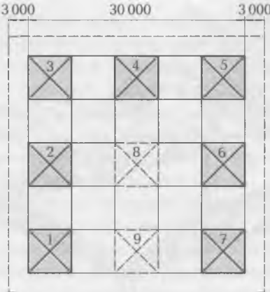
Рис. 9.13. Схема монтажа блоков лесов
