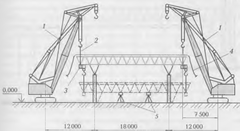
Рис. 10.3. Схема монтажа блока покрытия двумя кранами:
