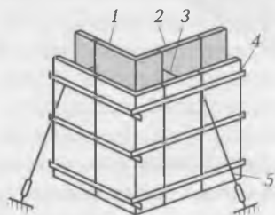
Рис. 11.5. Опалубка угла стен из крупноразмерных щитов: 1 — угловой щит; 2 — основной щит; 3 — стяжной болт; 4 — схватка; 5 — расчалка с фаркопом
