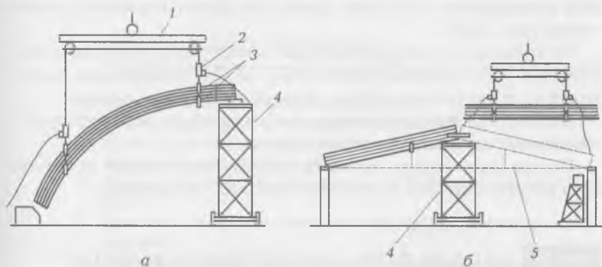
Рис. 13.4. Монтаж арок:
