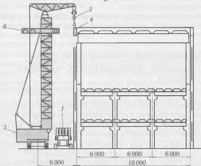
Рис. 9.4. Схемы монтажа стеновых панелей многоэтажных зданий самоходными кранами: a — со стреловым оборудованием; b — с башенно-стреловым оборудованием; 1 — кассеты с панелями; 2 — монтажный кран; 3 — строп; 4 — монтируемая стеновая панель; 5 — базовая машина; 6 — выдвижная люлька (площадка)
