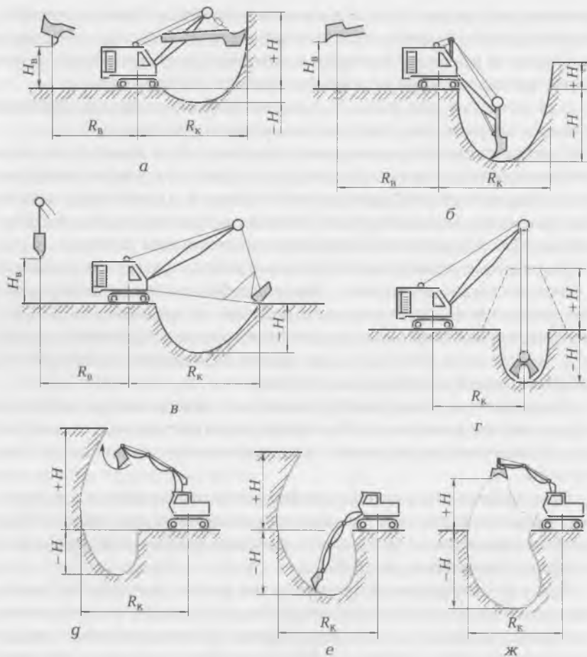
Рис. 4.7. Профили экскаваторных забоев с различным рабочим оборудованием: а — прямая лопата с канатным управлением рабочим оборудованием; б — обратная лопата; в — драглайн; г — грейфер; д — профиль забоя прямой лопаты с гидравлической системой управления; е — профиль забоя обратной лопаты; ж — грейфер; +H — высота копания; -H — глубина копания; H_0 — высота выгрузки; R_0 — радиус выгрузки; R_k — радиус копания
