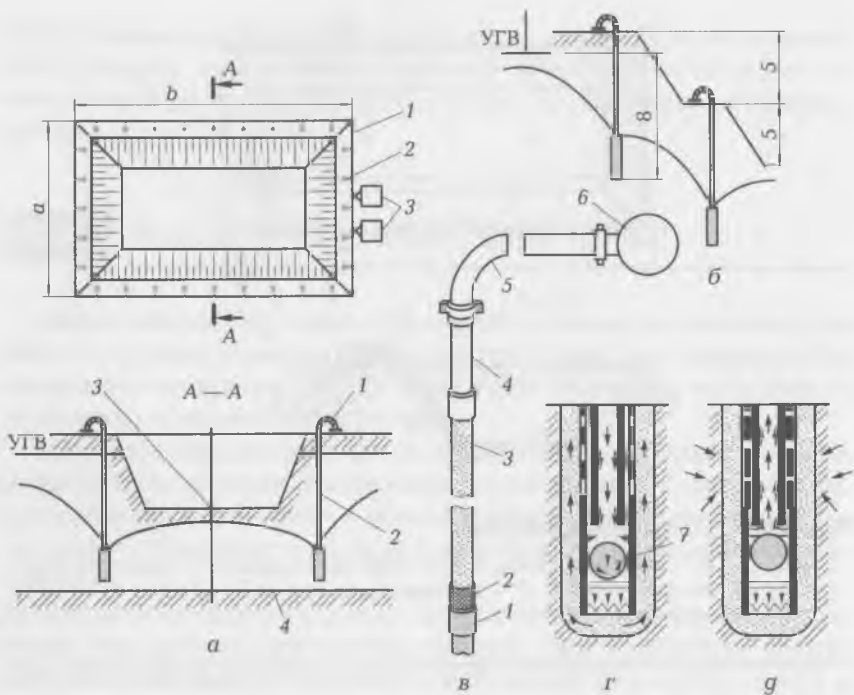
Рис. 4.4. Схема водопонижения легкими иглофильтровыми установками: а — план котлована с одноярусным расположением иглофильтров: 1 — коллектор; 2 — иглофильтр; 3 — вакуумный насос; 4 — водоупор; б — двухярусное расположение иглофильтров; в — схема иглофильтра: 1 — наконечник иглофильтра; 2 — фильтровая сетка; 3 — фильтровое перфорированное звено; 4 — надфильтровая труба; 5 — гибкий соединительный рукав; 6 — коллектор; 7 — шаровый клапан; г — схема движения воды при погружении иглофильтра; д — схема движения воды при откачке грунтовой воды (размеры указаны в м)
