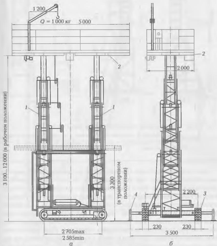
Рис. 6.25. Подмости выдвижные самоходные:
