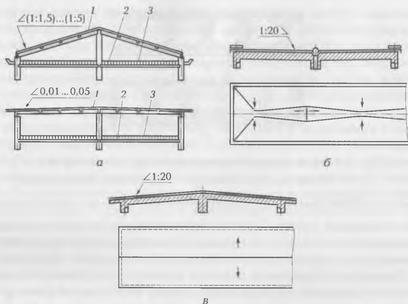
Рис. 1.9. Сборные железобетонные покрытия:
