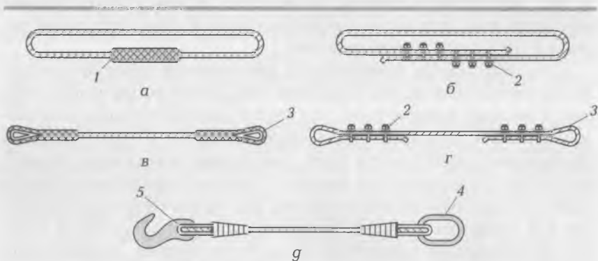
Рис. 6.7. Стropы универсальные:
