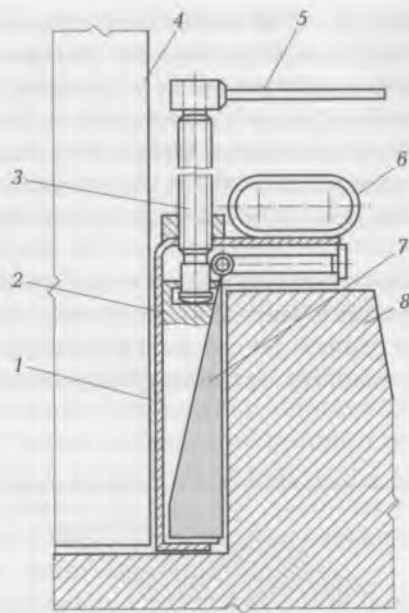
Рис. 6.19. Инвентарный клиновой вкладыш:
