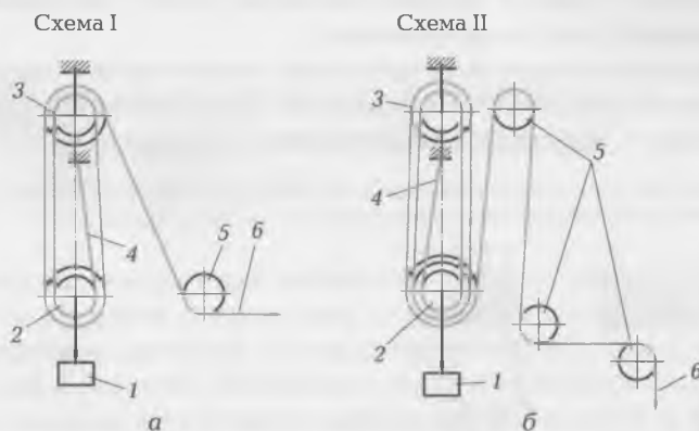
Рис. 6.15. Полиспаст:
