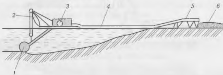
Рис. 4.14. Схема работы землесосного снаряда:
