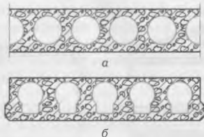
Рис. 1.7. Сборные железобетонные многопустотные настилы: а — с круглыми пустотами; б — с вертикальными пустотами
