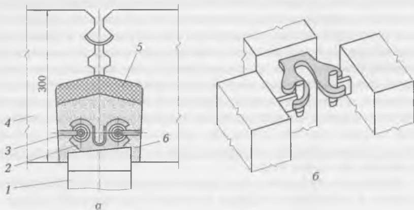
Рис. 9.9. Замковое соединение панелей:
