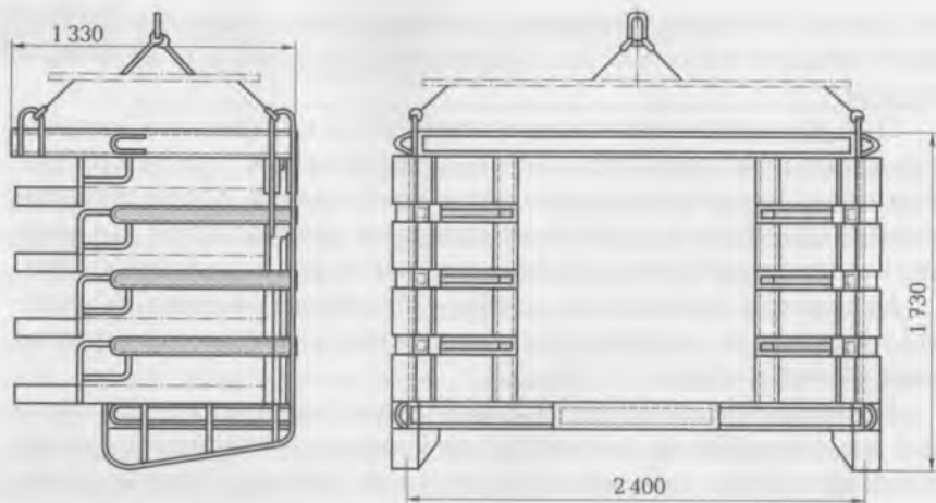
Рис. 5.2. Контейнер грузоподъемностью 3 220 кг для перевозки и монтажа четырех балконных плит
