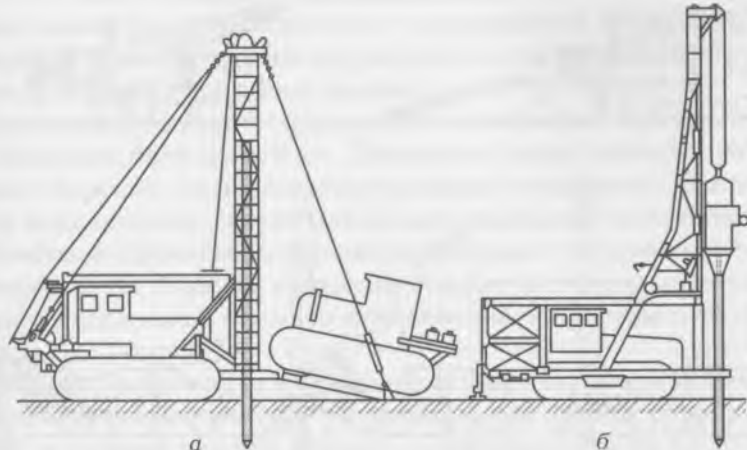
Рис. 8.12. Схема агрегатов для погружения свай методом вдавливания:
