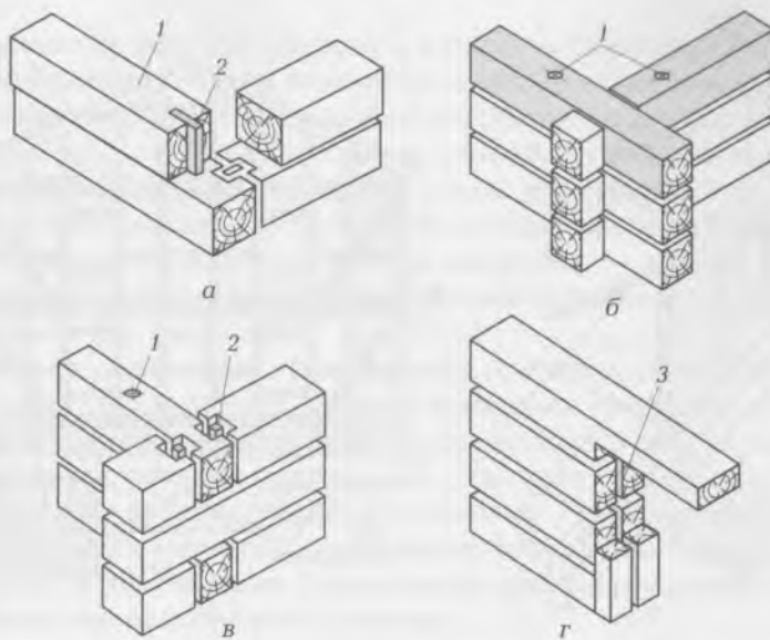
Рис. 13.2. Сборка стен зданий из брусьев:
