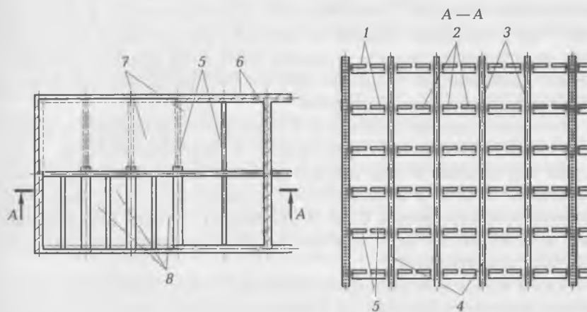
Рис. 1.12. Каркас здания с неполной каркасной системой:
