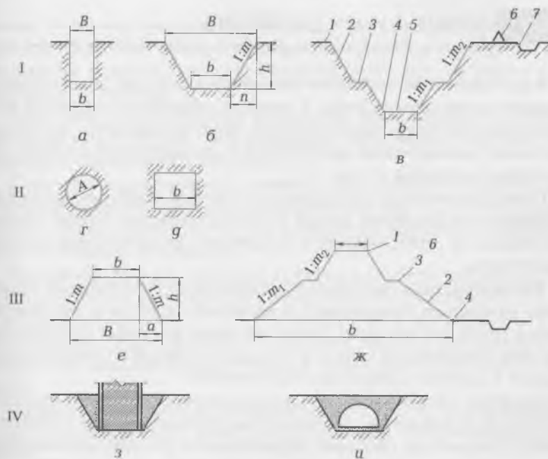
Рис. 4.1. Виды земляных сооружений:
