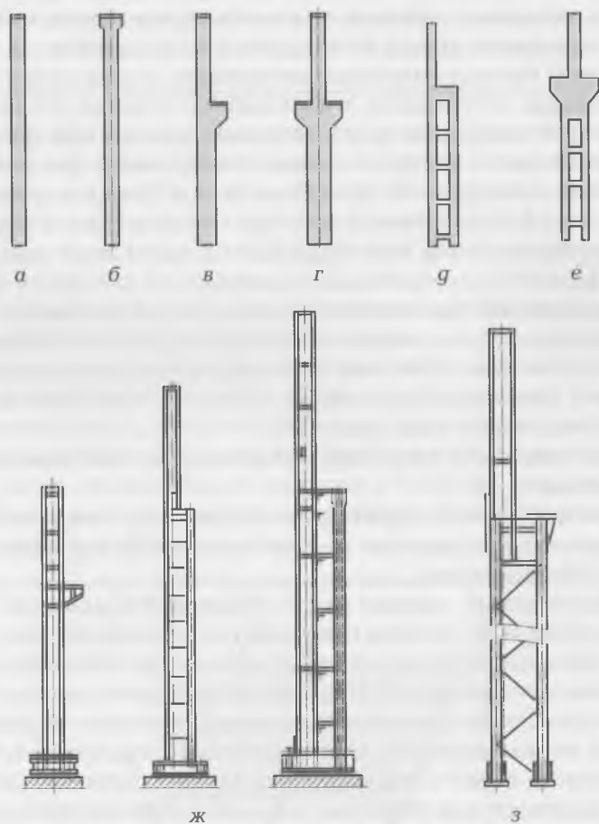
Рис. 1.6. Железобетонные (а—е) и металлические (ж,з) колонны:
