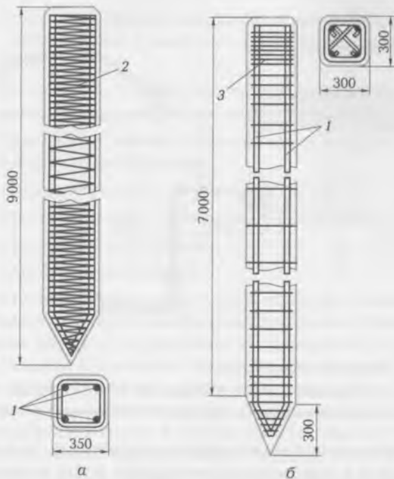
Рис. 8.7. Железобетонные сваи:
