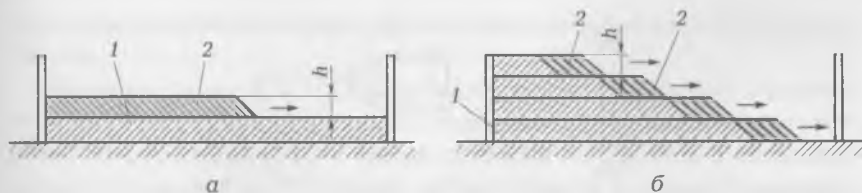
Рис. 11.13. Укладка бетонной смеси:
