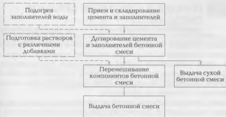
Рис. 11.12. Технологическая схема приготовления бетонной смеси
