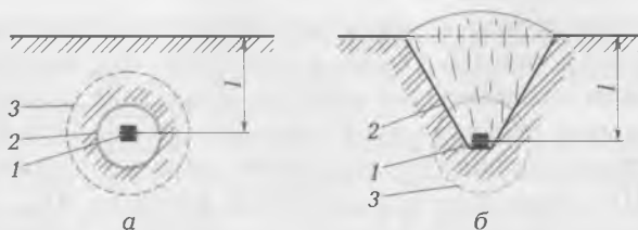
Рис. 4.19. Схемы действия взрыва на окружающую среду:
