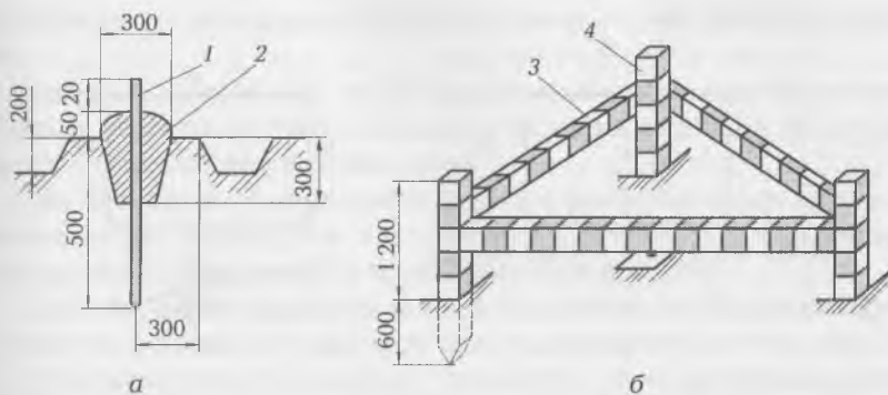
Рис. 3.2. Геодезический знак (а) и ограждение геодезического знака (б):
