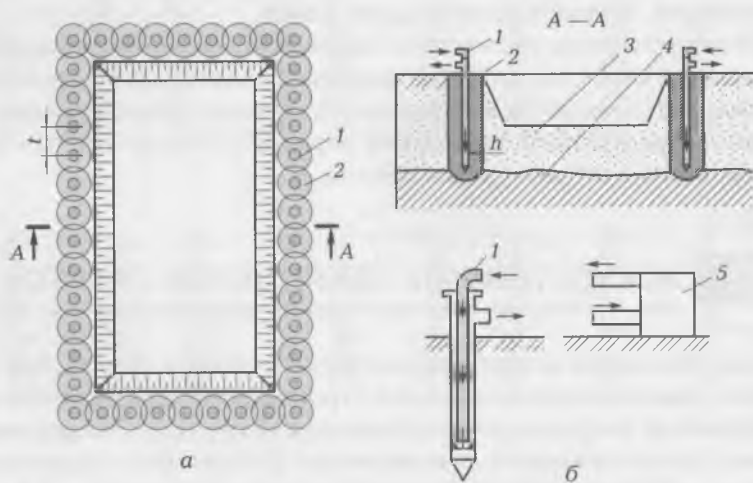
Рис. 4.6. Схема искусственного замораживания грунтов: а — план котлована с размещением замораживающих колонок; б — схема замораживающей колонки; 1 — замораживающая колонка; 2 — мерзлый грунт; 3 — талый грунт; 4 — водоупор; 5 — холодильная машина
