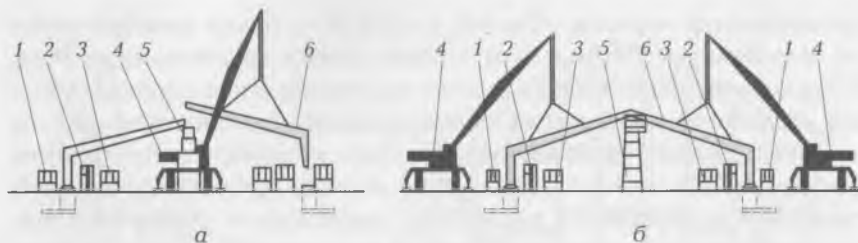
Рис. 13.5. Схема монтажа деревянных конструкций:
