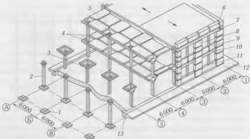
Рис. 1.13. Многоэтажное здание с безбалочными конструкциями перекрытий: 1 — фундамент; 2 — колонна; 3 — капитель; 4 — надколонная плита; 5 — пролетная плита; 6 — карнизные блоки; 7, 10 — перемычные блоки; 8 — простеночные блоки; 9 — подоконные блоки; 11 — цокольные блоки; 12 — отводка; 13 — фундаментная балка
