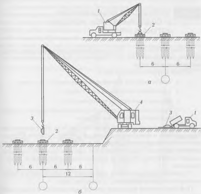
Рис. 8.15. Схема технологического процесса устройства монолитного ростверка: а — установка арматурно-опалубочных блоков; б — бетонирование ростверков; 1 — автомобильный кран; 2 — арматурно-опалубочный блок; 3 — поворотная бадейка; 4 — гусеничный кран; 5 — автомашина (размеры указаны в м)
