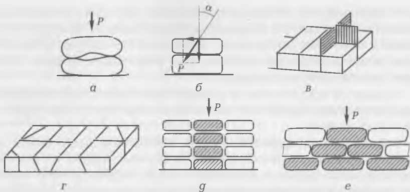
Рис. 12.2. Правила разрезки каменной кладки:
