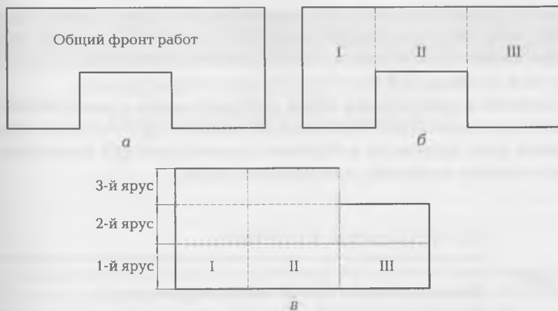
Рис. 2.5. Разбивка общего фронта работ:
