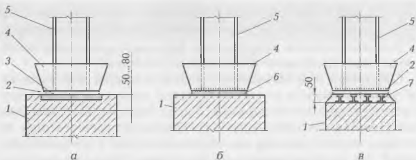
Рис. 10.1. Схемы опирания металлических колонн на фундаментах: а — на заранее выверенные стальные плиты с верхней фрезерованной поверхностью; б — непосредственно на фундамент, возведенный до проектной отметки установки колонны; в — на заранее установленные опорные детали; 1 — железобетонный фундамент; 2 — бетон подливки; 3 — опорная плита; 4 — башмак; 5 — колонна; 6 — опорная плита башмака; 7 — рельсы
