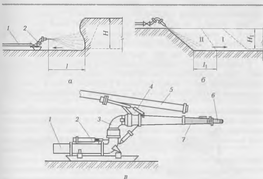
Рис. 4.13. Схема разработки грунта гидромонитором:
