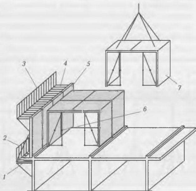
Рис. 11.7. Схема установки щитов объемно-переставной (туннельной) опалубки: 1, 4 — консольные подмости; 2, 3 — ограждения; 5 — боковой щит; 6 — механический домкрат; 7 — блок объемно-переставной опалубки
