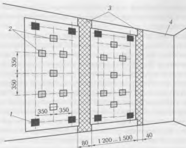
Рис. 16.7. Приклеивание листов сухой штукатурки:
