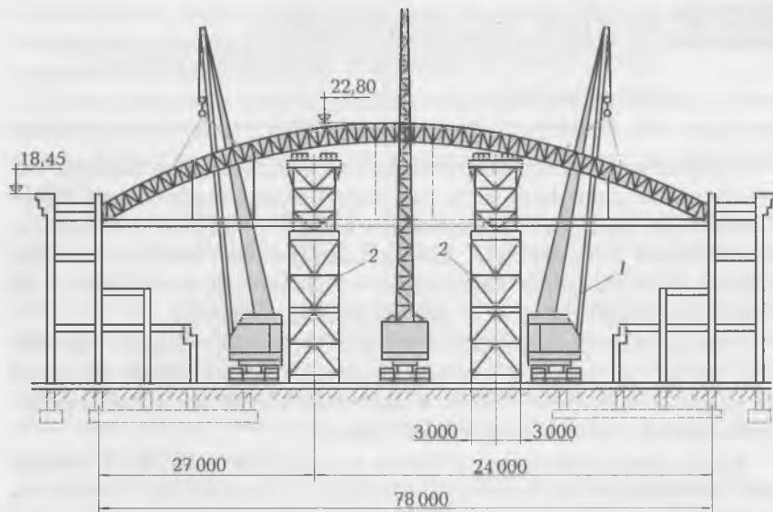
Рис. 10.2. Монтаж арочного большепролетного покрытия:
