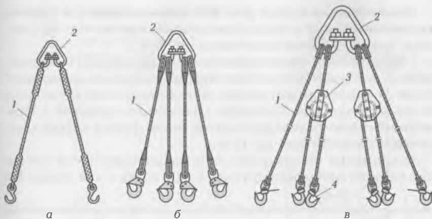
Рис. 6.8. Многоветвевые стропы:
