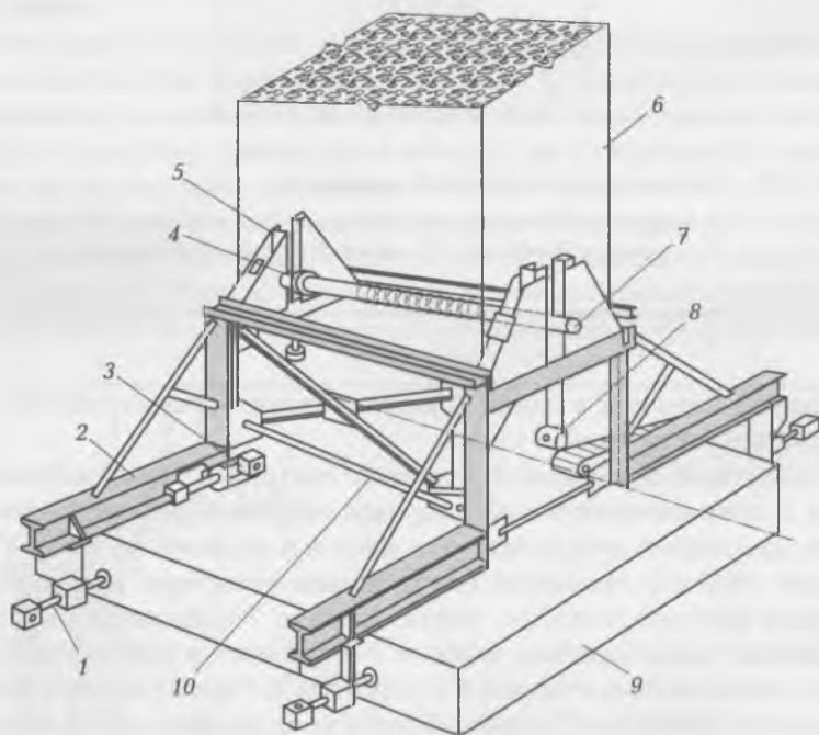
Рис. 6.20. Кондуктор для выверки и временного закрепления колонн:
