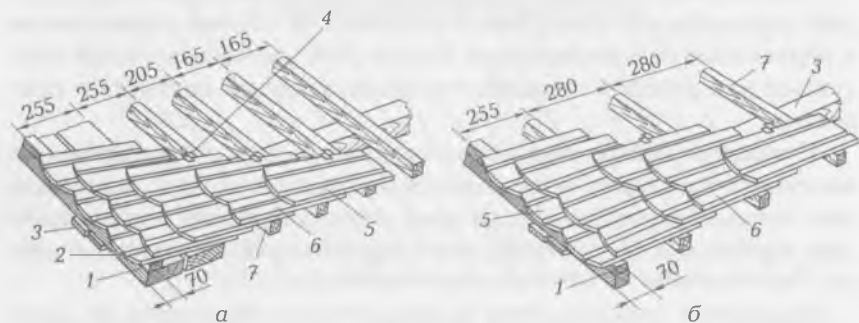
Рис. 14.5. Покрытие крыши плоской ленточной черепицей:
