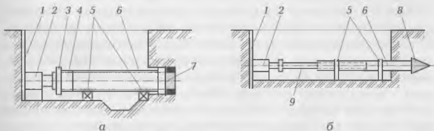
Рис. 4.16. Схемы закрытых (бестраншейных) способов прокладки трубопроводов:
