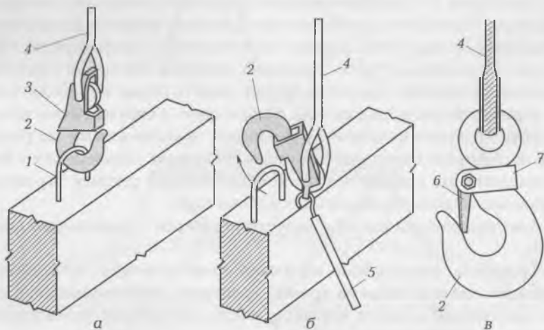
Рис. 6.12. Грузозахватные устройства с дистанционной отцепкой крюка, положение крюка: а — после строповки; б — после расстроповки; в — крюк с предохранительным устройством; 1 — монтажная петля; 2 — крюк; 3 — карабин; 4 — строп; 5 — тяга; 6 — отжимная пружина; 7 — скоба с болтом
