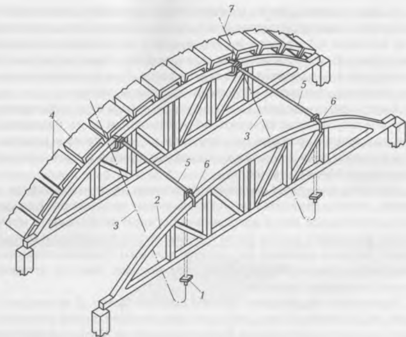
Рис. 6.21. Временное закрепление ферм инвентарными распорками:
