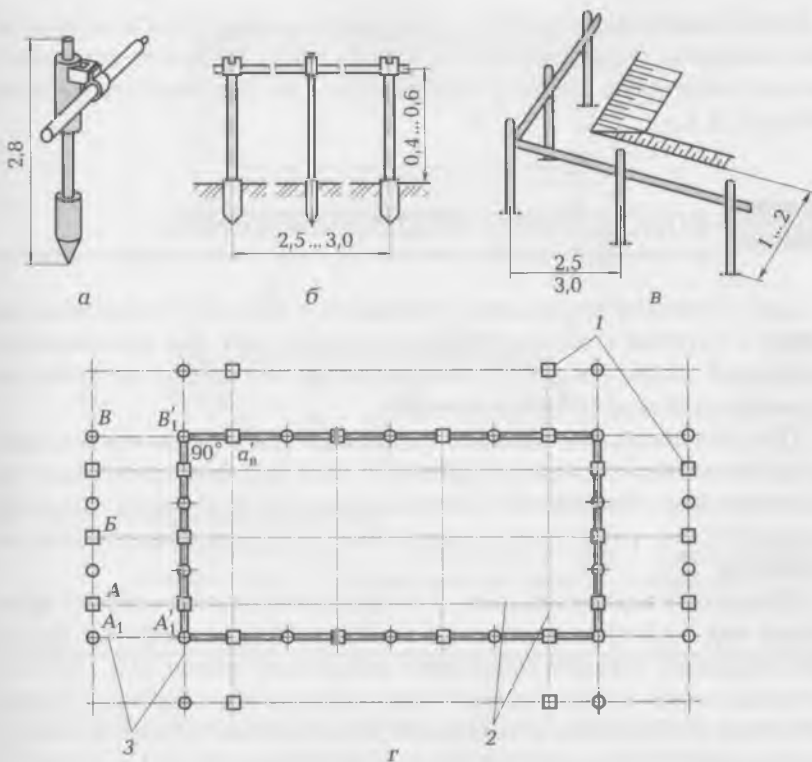
Рис. 4.2. Элементы геодезической разбивки земляного сооружения: а — инвентарная металлическая стойка обноски; б — схема закрепления осей; в — схема расположения обноски; г — план разбивки котлована: 1 — опорные знаки; 2 — основные оси здания; 3 — установленные оси обноски (размеры указаны в м)
