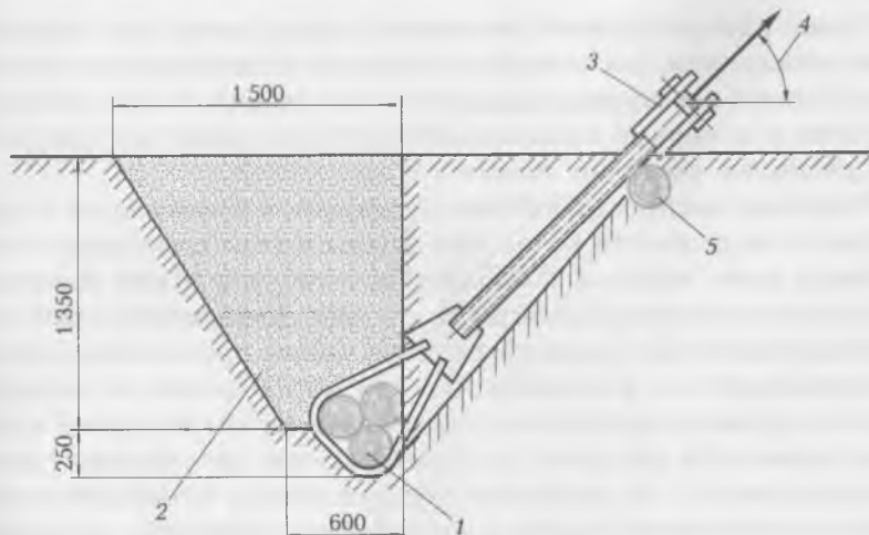
Рис. 6.17. Заглубленный горизонтальный якорь:
