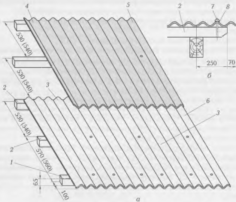
Рис. 14.4. Устройство кровли из волнистых асбоцементных листов: а — начальная стадия для укладки листов; б — поперечный разрез фронтового свеса; 1 — карнизный брусок; 2 — обрешетка; 3 — сливной лист; 4 — рядовой лист; 5 — фронтовый лист; 6 — угловой лист; 7 — гвоздь; 8 — резиновая шайба
