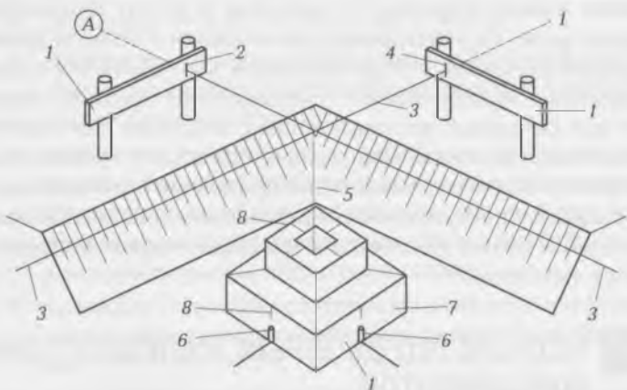
Рис. 8.1. Геодезическая разбивка столбчатых фундаментов: 1 — обноска; 2, 8 — риски; 3 — проволока; 4 — положение разбивочных осей на обноске; 5 — отвес; 6 — колышки-фиксаторы; 7 — фундамент
