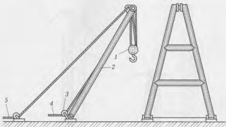
Рис. 6.5. Шевр:
