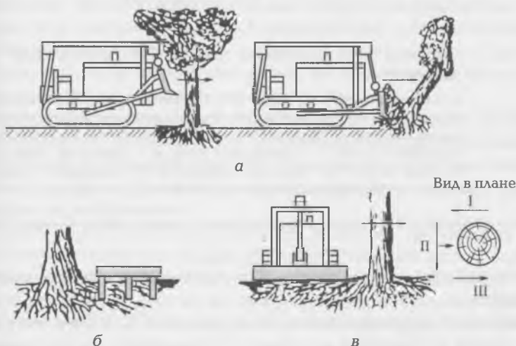
Рис. 3.4. Валка деревьев:
