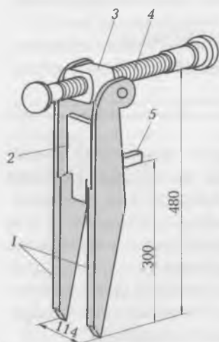
Рис. 6.18. Металлический клин для закрепления колонн:
