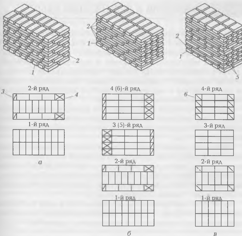
Рис. 12.3. Системы перевязки при кладке стен толщиной в два кирпича:
