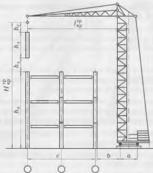
Рис. 6.6. Схема для определения параметров башенного крана
