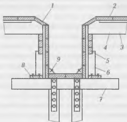
Рис. 11.3. Опалубка балок:
