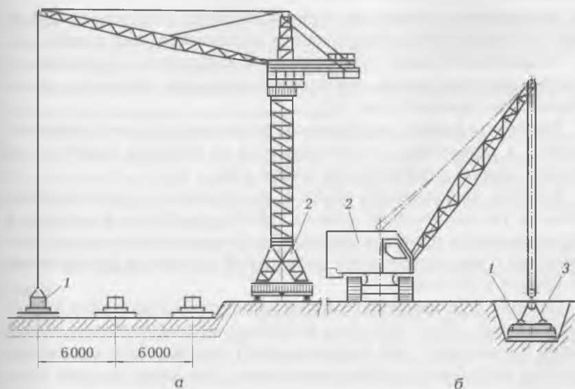
Рис. 8.2. Монтаж сборных фундаментов: а — башенными кранами; б — гусеничными кранами; 1 — сборный элемент фундамента; 2 — кран; 3 — строп
