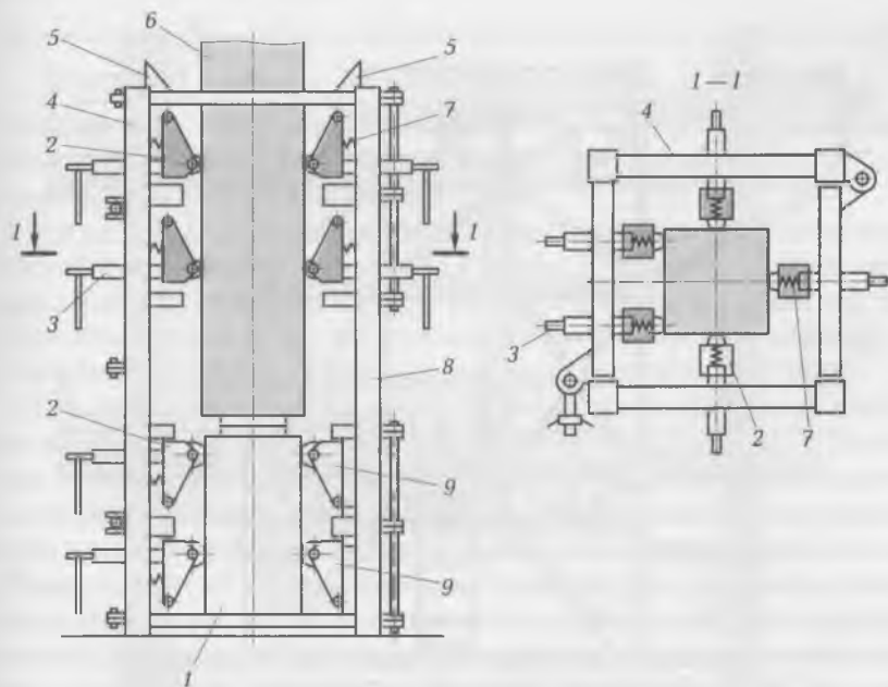
Рис. 6.22. Одиночный кондуктор для установки и выверки колонн многоэтажных зданий:
