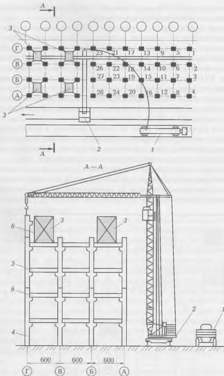
Рис. 9.3. Схема организации возведения многоэтажного каркасного здания: 1 — транспортные средства; 2 — кран; 3 — кондуктор; 4 — колонна; 5 — балки; 6 — плиты перекрытия (1...28 — очередность монтажа колонн)
