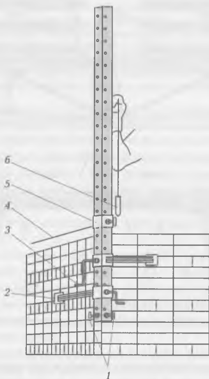
Рис. 12.9. Порядовка угловая:
