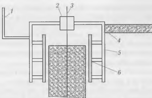
Рис. 11.8. Схема скользящей опалубки:
