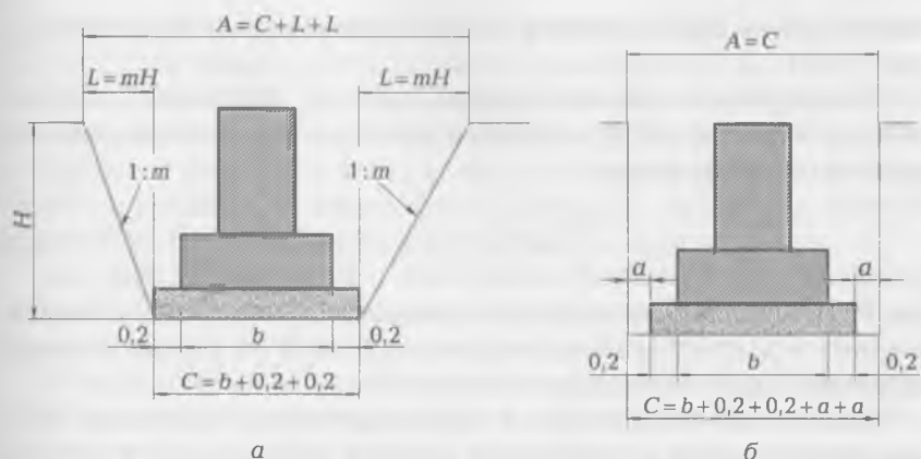
Рис. 4.12. Определение размеров земляного сооружения по дну C и верху A :
