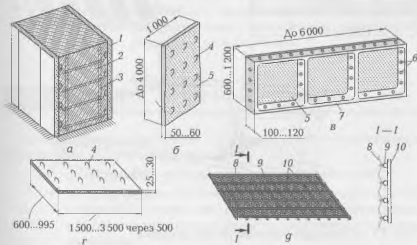
Рис. 11.9. Несъемная опалубка:
