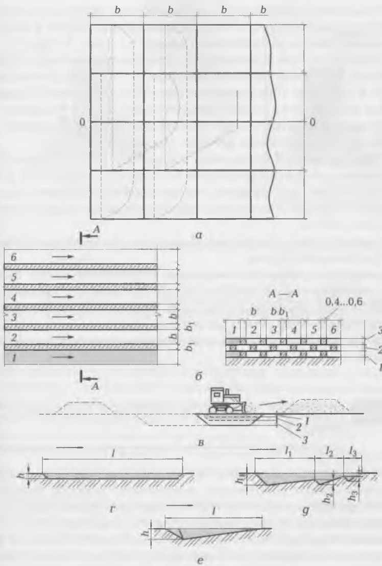
Рис. 4.11. Схемы работы бульдозера:
