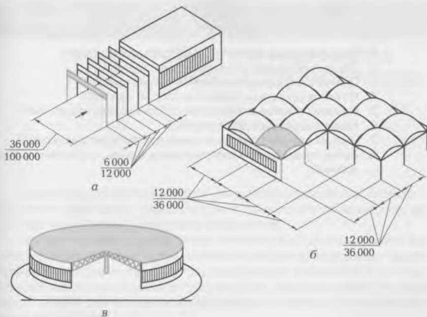
Рис. 1.14. Типы зданий в зависимости от расположения опор: а — пролетные; б — ячейковые; в — зальные с центральной опорой
