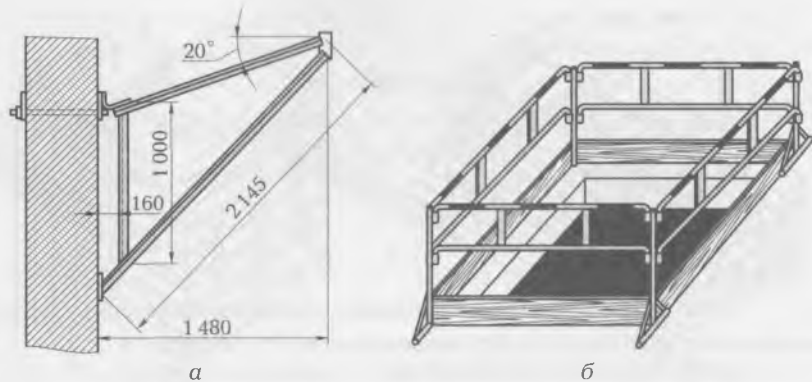
Рис. 12.14. Инвентарные приспособления:
