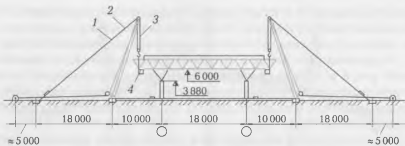
Рис. 10.4. Подъем блока размером 30×30 м шеврами:
