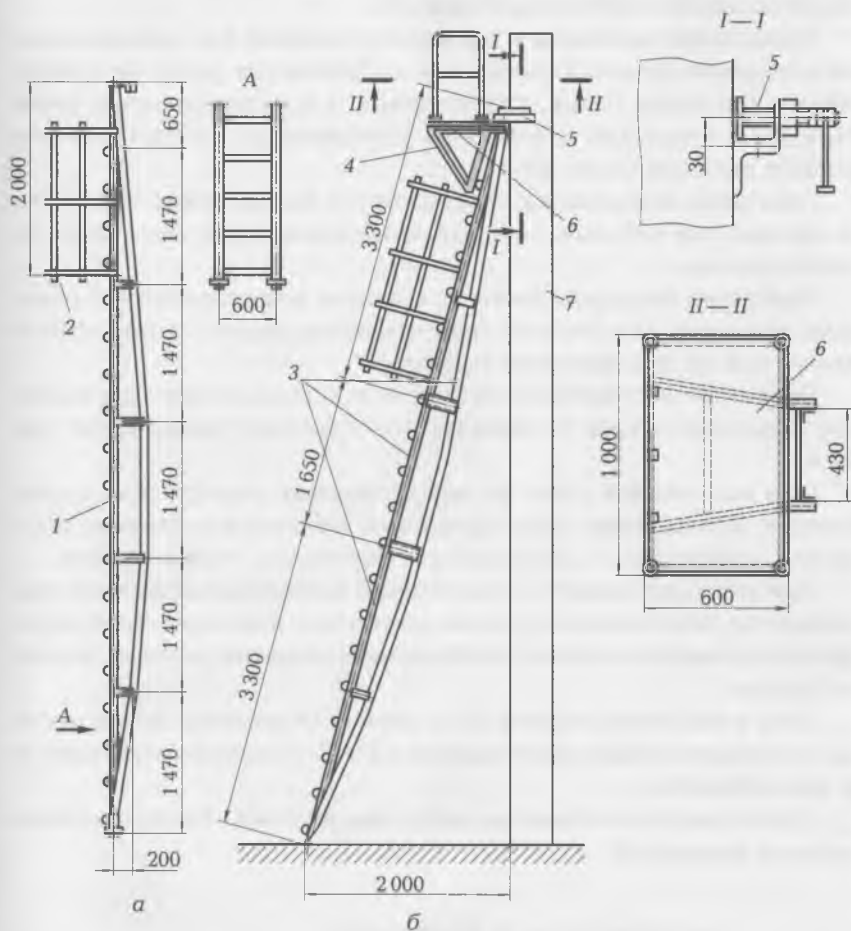
Рис. 6.27. Приставные секционные лестницы:
