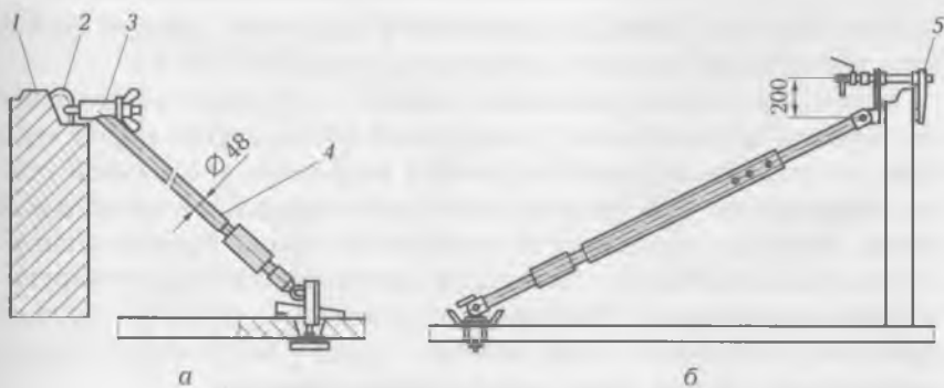
Рис. 9.8. Схемы временного крепления стеновых панелей с помощью подкосов: а — захватной головкой бесструбцинного подкоса; б — струбцинным подкосом; 1 — панель; 2 — монтажная петля; 3 — захватная головка; 4 — подкос; 5 — струбцина
