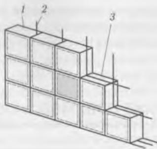
Рис. 16.1. Остекление из стеклоблоков:
