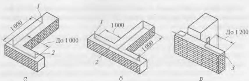
Рис. 12.12. Усиление кладки стальными связями:
