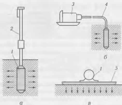
Рис. 11.14. Типы вибраторов и схемы передачи колебаний бетонной смеси:
