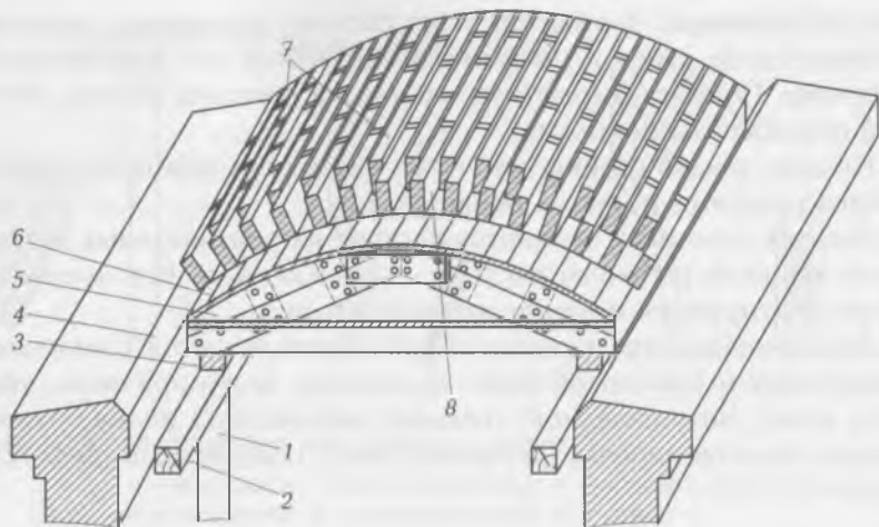
Рис. 12.10. Кладка сводов:
