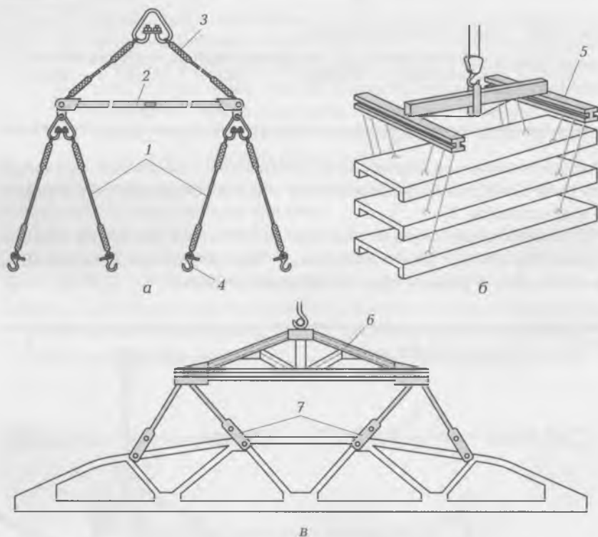
Рис. 6.10. Траверсы:
