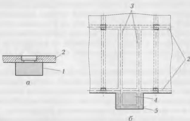
Рис. 1.5. Балкон (а) и эркер (б): 1 — консольная плита; 2 — наружная стена; 3 — балка перекрытия; 4 — эркер; 5 — ригель
