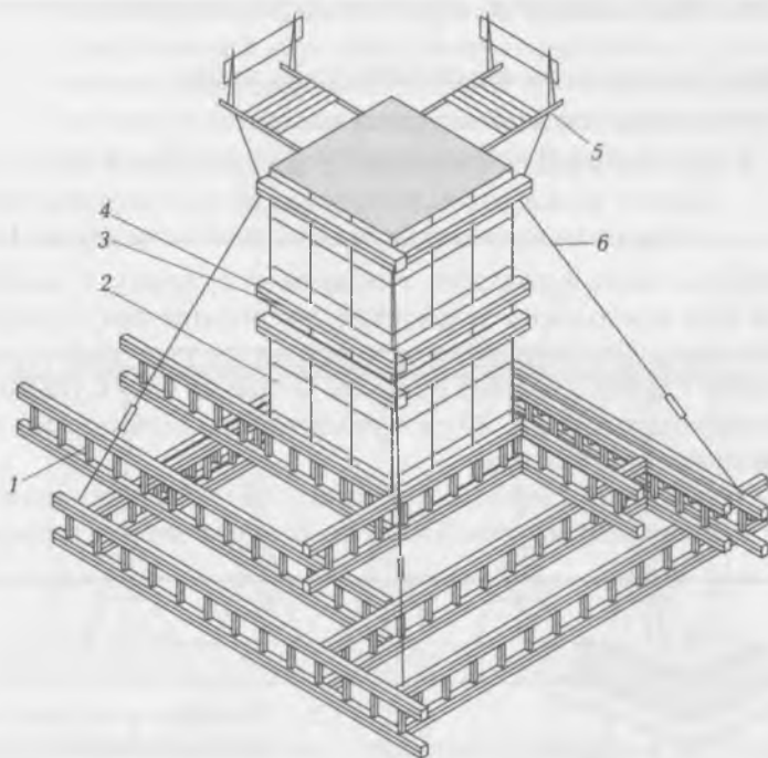
Рис. 11.4. Стальная опалубка ступенчатого фундамента:
