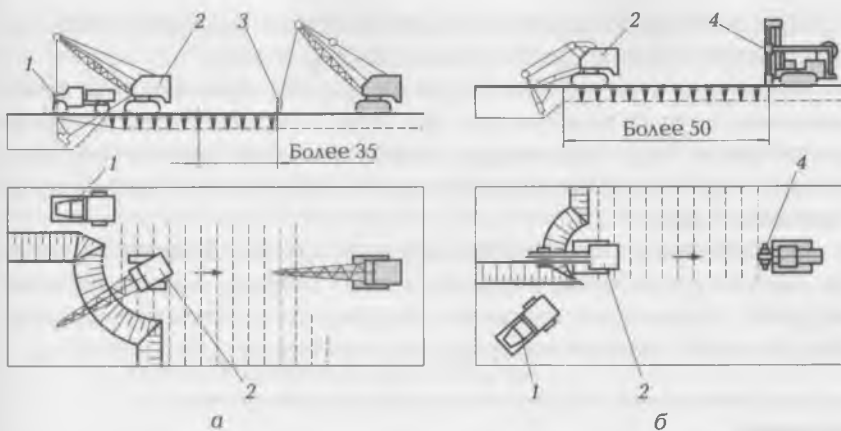
Рис. 4.21. Схемы разработки мерзлых грунтов с предварительным рыхлением: а — рыхление клин-молотом; б — рыхление тракторным виброклиновым рыхлителем; 1 — автосамосвал; 2 — экскаватор; 3 — клин-молот; 4 — виброклин (размеры указаны в м)
