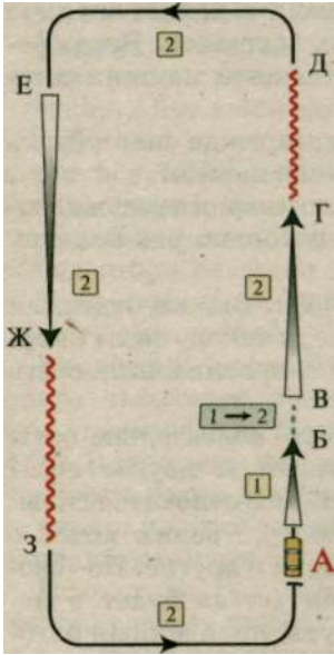
Рис. 44. Разгон, торможение и поворот на второй •передаче: А - старт и остановка; А-Б - разгон; 1→2 (Б-В) переключение с первой передачи на вторую; В-Г и Е-Ж - разгон; Г-Д и Ж-3 - торможение; Д-Е и 3-А - два поворота
