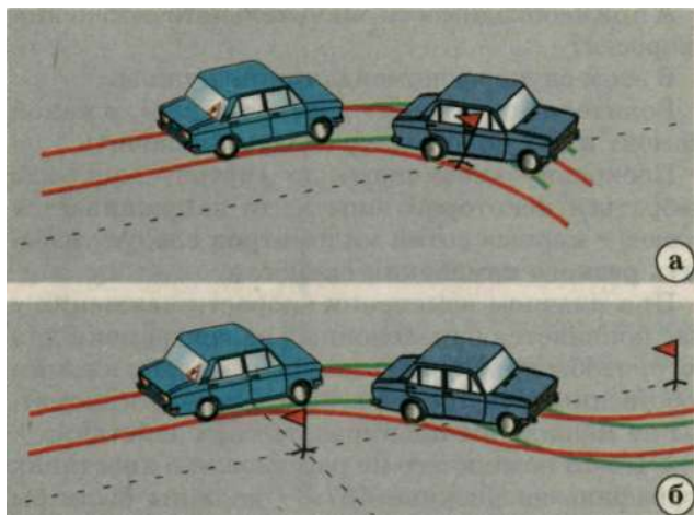
Рис. 42. Траектории движения передних и задних колес
